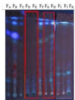
Gambar 6. Profil noda fraksi A, B, C, D, E, F, G, H, I, J, dan K dengan pengembang n-heksana: diklorometana 2:1 di bawah lampu UV 365 nm
