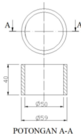
Gambar 2. Bentuk dan Dimensi Shell RSB
