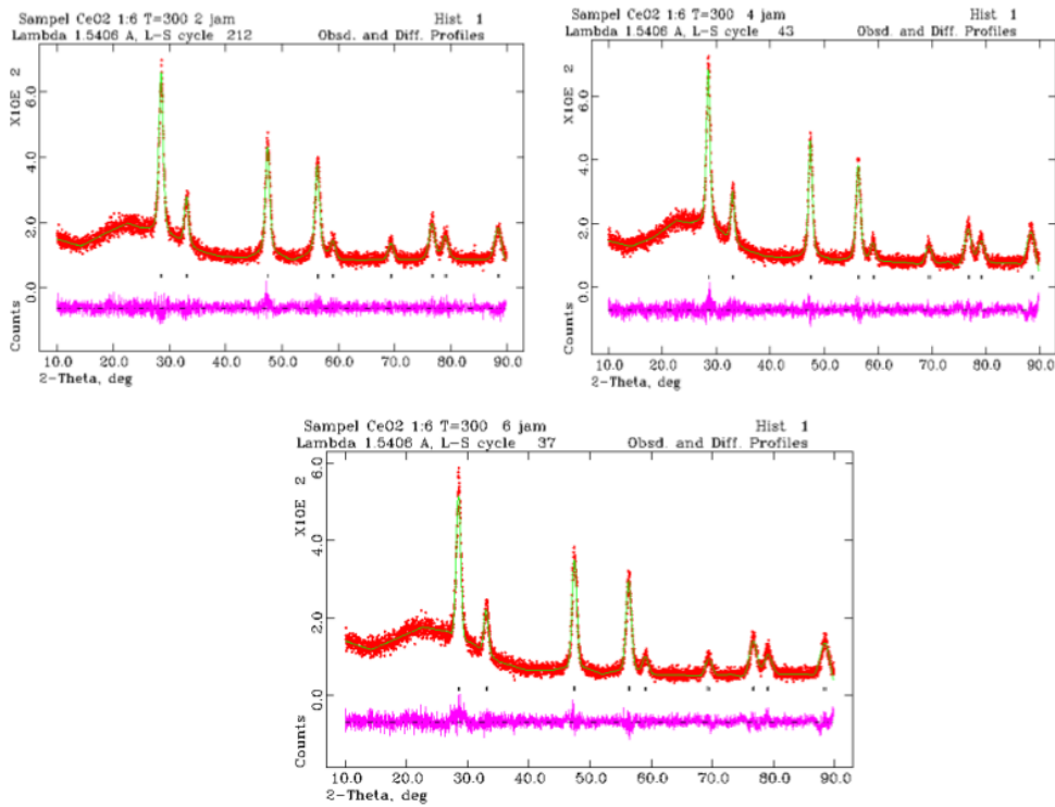
Gambar 2. Hasil pencocokan pola difraksi sinar-x nanokristalin CeO_2 yang dikalsinasi pada temperatur 300^\circ C selama (a) 2 jam, (b) 4 jam dan (c) 6jam
