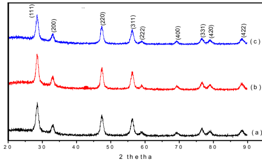
Gambar 1. Pola Difraksi sinar-x nanokristalin CeO_2 yang dikalsinasi pada temperatur 300^\circ C selama (a) 2 jam, (b) 4 jam dan (c) 6 jam
