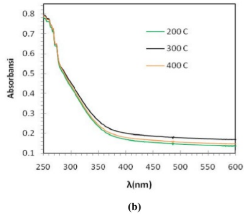
dan (b) absorpsi nanopartikel cerium oxide yang dikalsinasi pada berbagai temperatur
