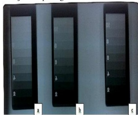
Gambar 3. Citra Radiograf Stepwedge pada Imaging Plate 35x43 cm, a) ekspos pertama, b) ekspos kedua dan c) ekspos ketiga
