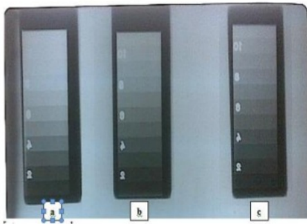
Gambar 1. Citra Radiograf Stepwedge pada Imaging Plate 18x24 cm, a) ekspos pertama, b) ekspos kedua dan c) ekspos ketiga
