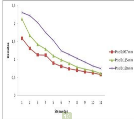
Gambar 4. Grafik densitas rata-rata dari masing-masing ukuran imaging plate
