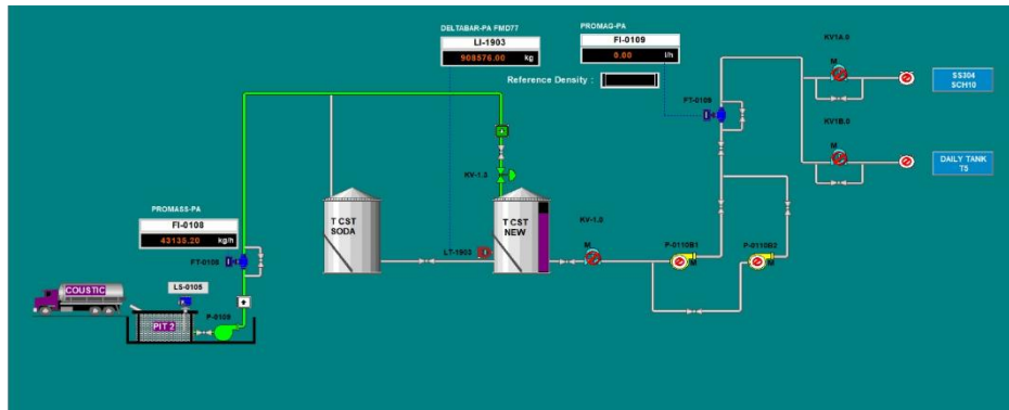
Gambar 4.19 Dokumentasi Pengambilan Data Flowmeter di SCADA
