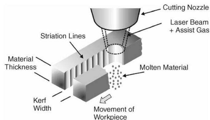
Gambar 2.2 Ilustrasi Proses Laser Cutting pada Material Logam (Abdel Ghany & Newishy, 2005)
