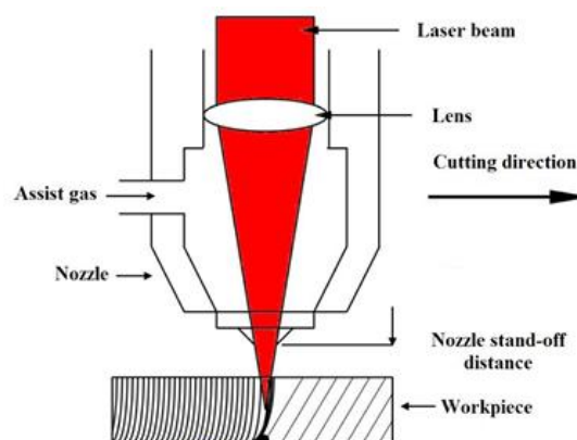
Gambar 2.8 Ilustrasi Pemotongan dengan Laser CO 2 (M., et al., 2016)
