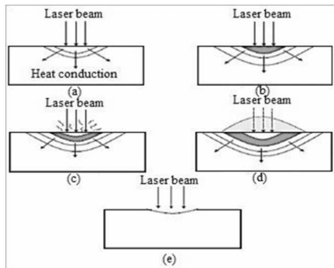
Gambar 2.5 Ilustrasi Efek yang terjadi Interaksi Laser dengan (a) pemanasan, (b) pelelehan permukaan, (c) penguapan permukaan, (d) pembentukan plasma, dan (e) ablasi
