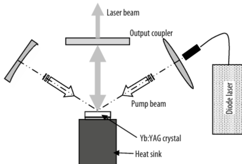
Gambar 2.9 Ilustrasi Pemotongan dengan Laser Diode (Steen & Mazumder 2010)
