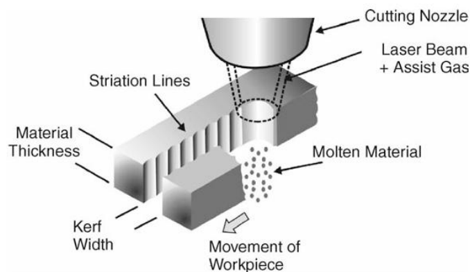
Gambar 2. 3 Ilustrasi Proses Laser Cutting pada Material Logam
