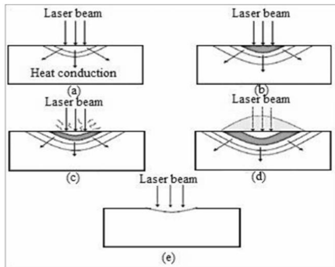
Gambar 2. 6 Ilustrasi Efek yang terjadi Interaksi Laser dengan
