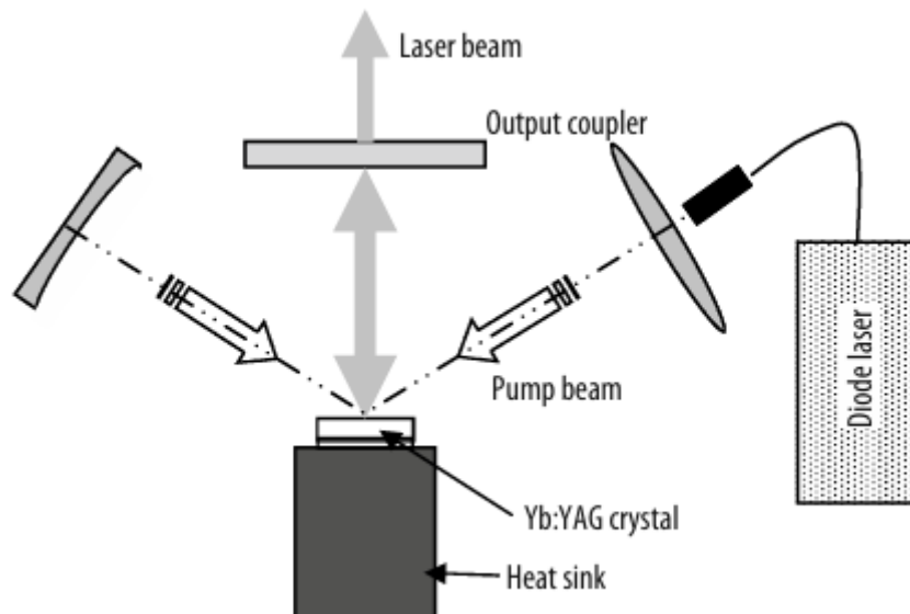
Gambar 2. 10 Ilustrasi Pemotongan dengan Laser Diode
