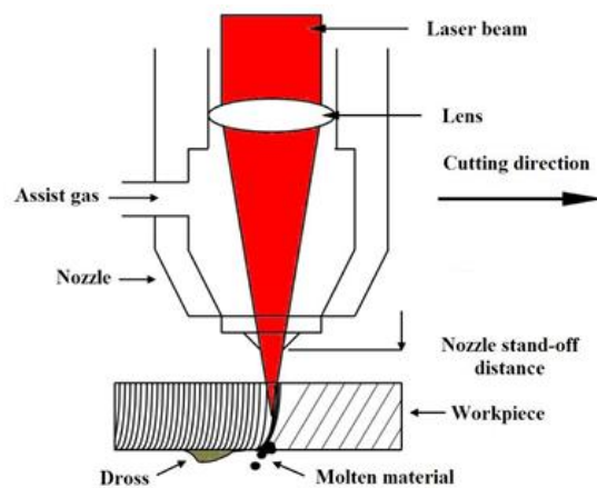
Gambar 2. 9 Ilustrasi Pemotongan dengan Laser CO 2
