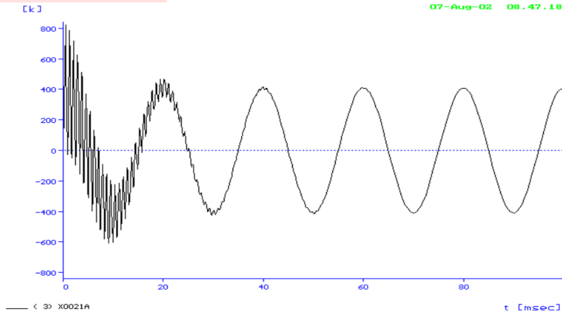
Gambar 2. Profil Surja Hubung di Ujung Saluran Transmisi 500 kV Ungaran-Pedan pada Saat Operasi Energized.
