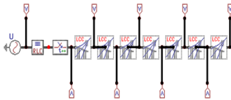
Gambar 1. Model Rangkaian untuk Simulasi
