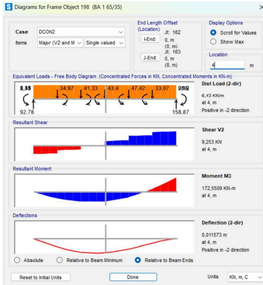
Gambar 4. 33 Output Momen Lapangan Arah Positif Balok BA1
