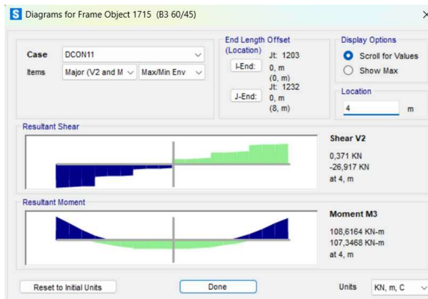
Gambar 4. 23 Output Momen Lapangan Arah Negatif Balok B3
