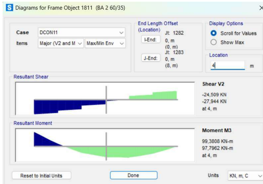
Gambar 4. 41 Output Momen Lapangan Arah Negatif Balok BA1
