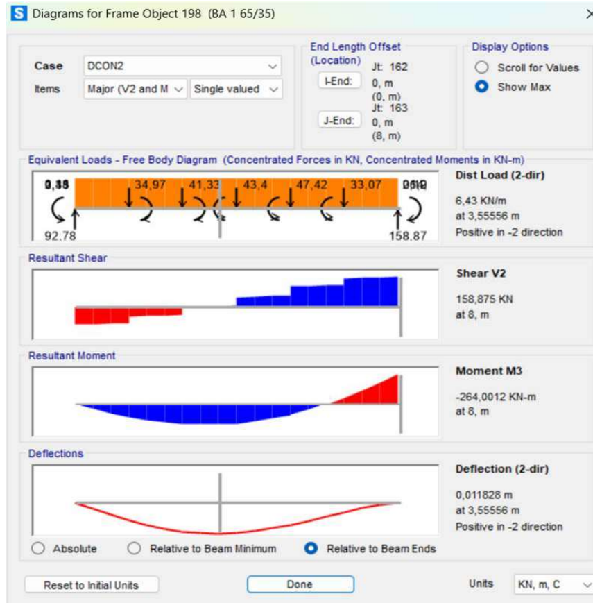
Gambar 4. 35 Output Gaya Geser Tumpuan Balok BA1
