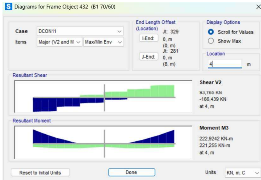
Gambar 4. 9 Output Gaya Geser Lapangan Balok B1
