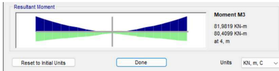
Gambar 4. 5 Output Momen Lapangan Arah Negatif Balok B1
