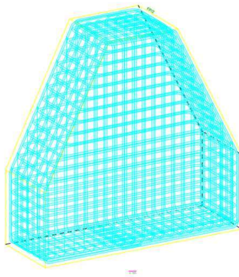
Gambar 4. 60 Detail Penulangan PileCap PC-2
