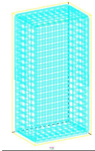
Gambar 4. 61 Detail Penulangan PileCap PC-3
