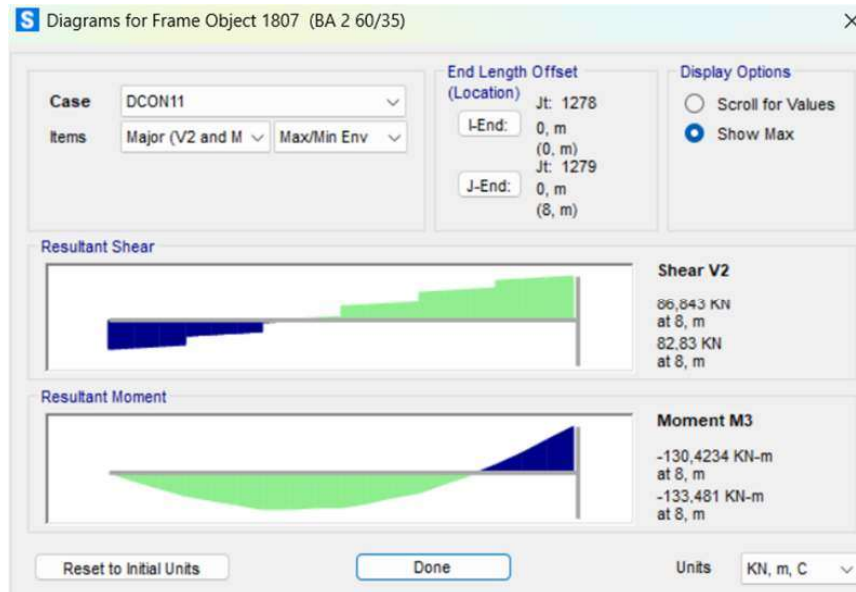
Gambar 4. 40 Output Momen Tumpuan Arah Positif Balok BA1
