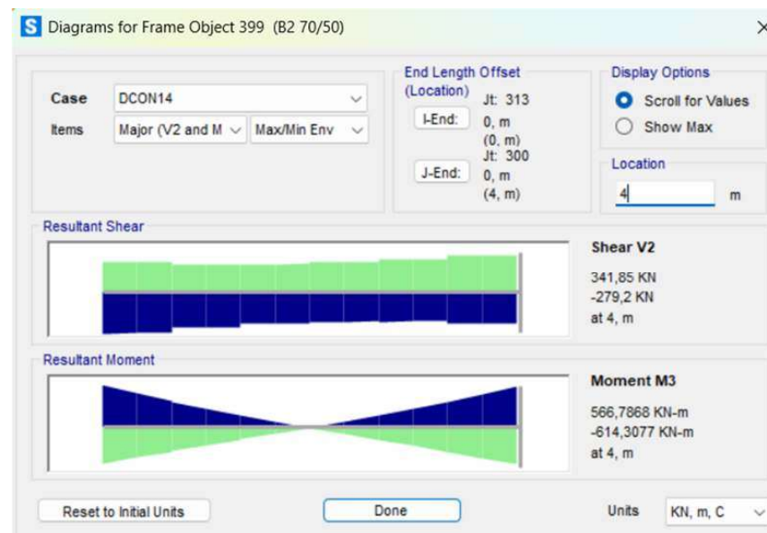
Gambar 4. 13 Output Momen Tumpuan Arah Positif Balok B2
