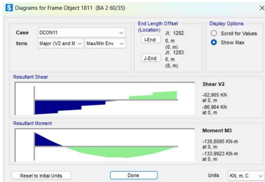
Gambar 4. 44 Output Gaya Geser Tumpuan Balok BA2
