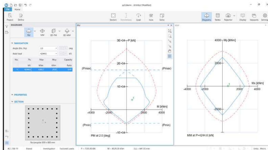
Gambar 4. 51 Diagram Interaksi Kolom K2 dengan aplikasi spColumn
