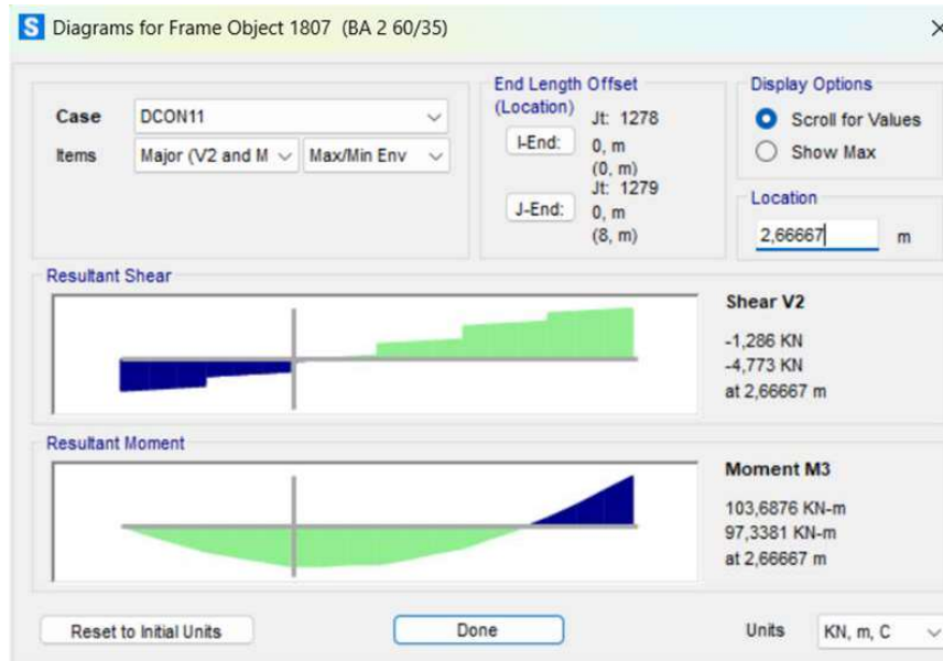
Gambar 4. 42 Output Momen Lapangan Arah Positif Balok BA1
