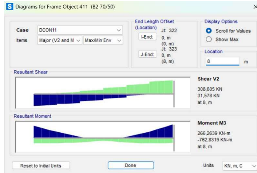
Gambar 4. 12 Output Momen Tumpuan Arah Negatif Balok B2
