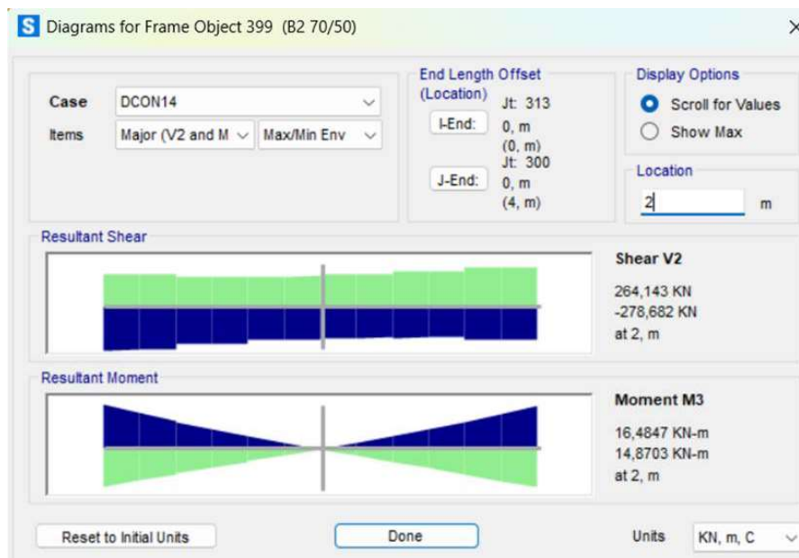
Gambar 4. 18 Output Gaya Geser Lapangan Balok B2
