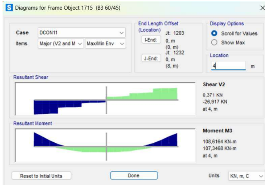
Gambar 4. 27 Output Gaya Geser Lapangan Balok B3
