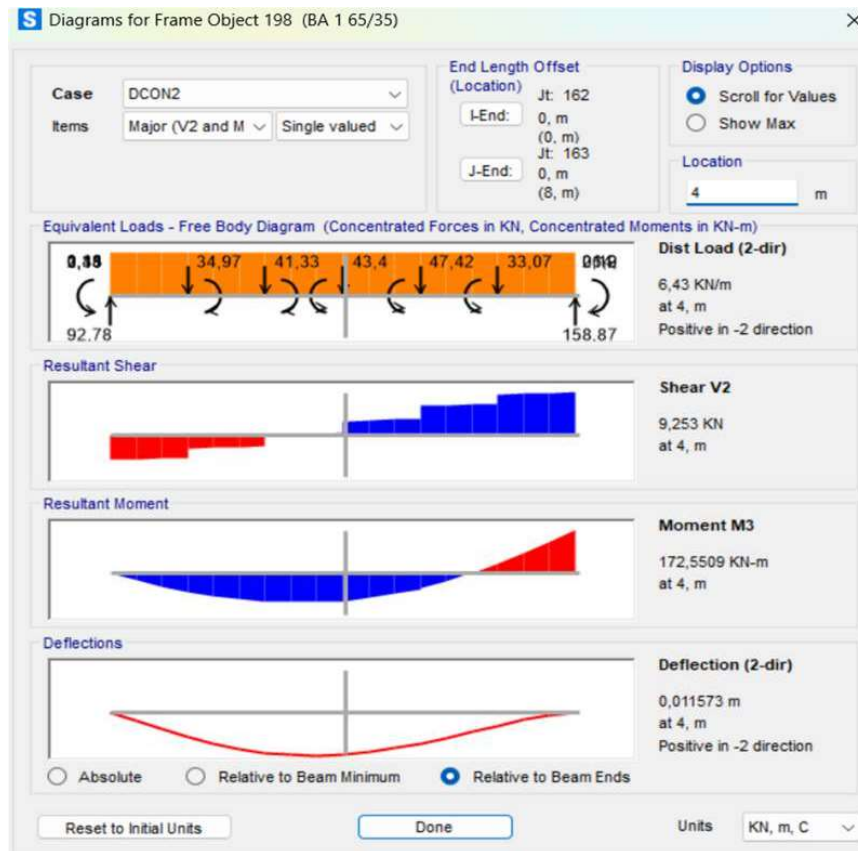
Gambar 4. 36 Output Gaya Geser Lapangan Balok BA1
