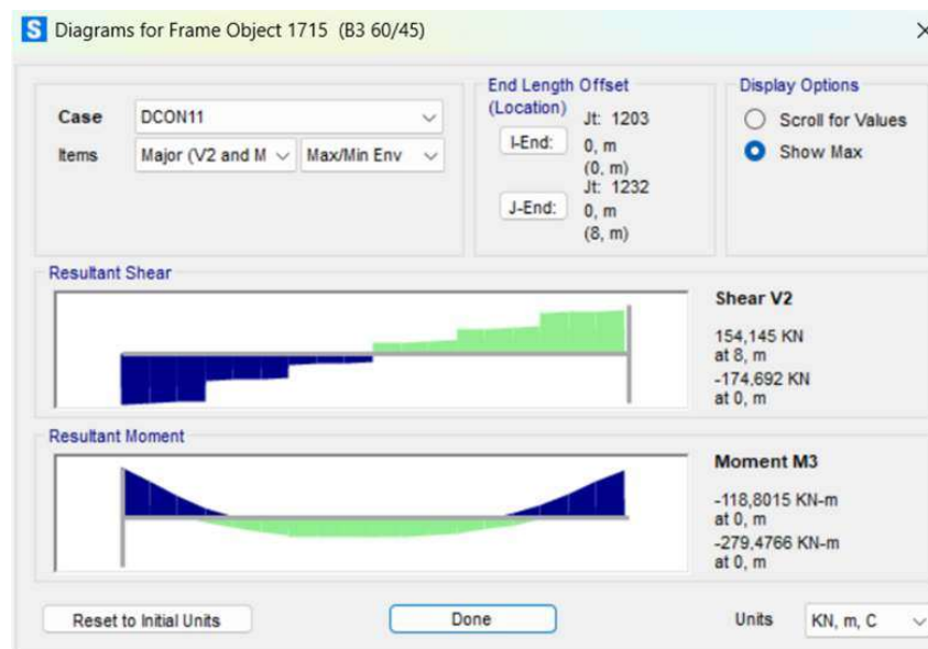
Gambar 4. 26 Output Gaya Geser Tumpuan Balok B3
