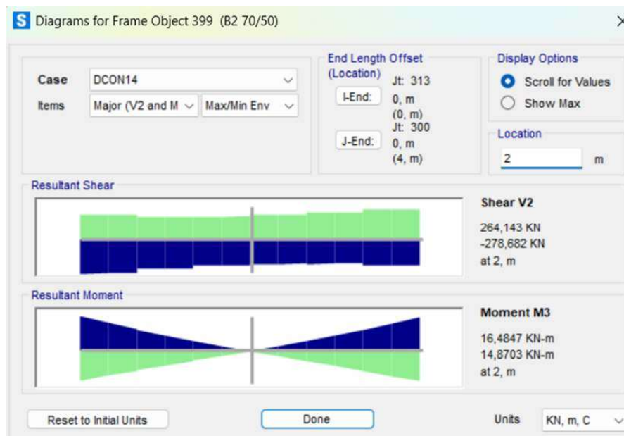
Gambar 4. 15 Output Momen Lapangan Arah Positif Balok B2
