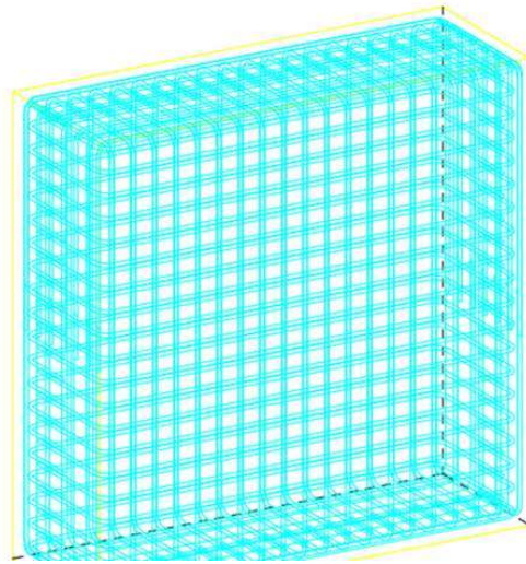
Gambar 4. 59 Detail Penulangan PileCap PC-1
