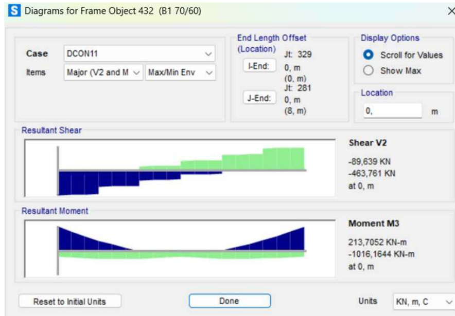
Gambar 4. 3 Output Momen Tumpuan Arah Negatif Balok B1
