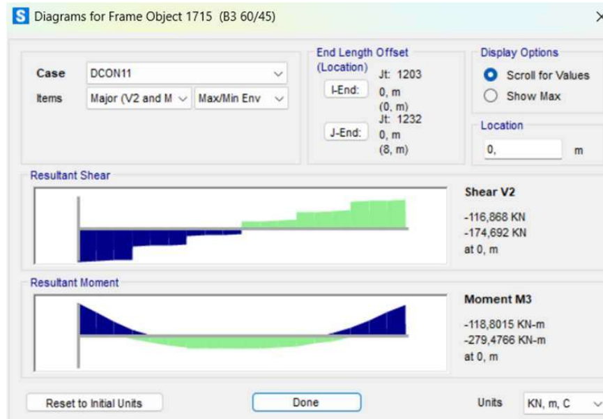
Gambar 4. 21 Output Momen Tumpuan Arah Negatif Balok B3
