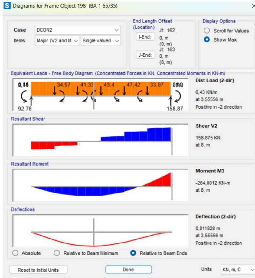
Gambar 4. 31 Output Momen Tumpuan Arah Positif Balok BA1
