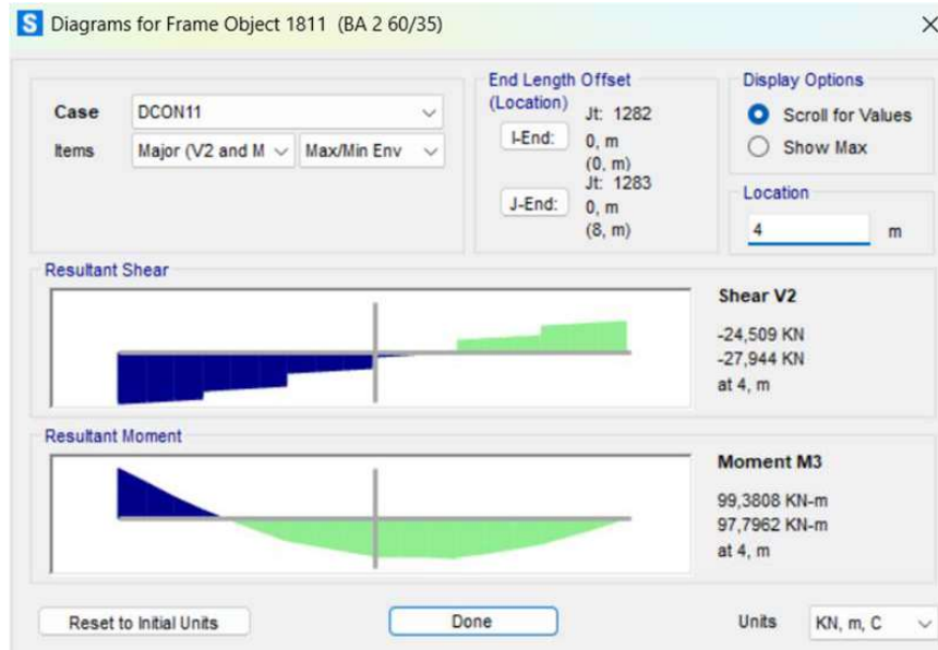
Gambar 4. 45 Output Gaya Geser Lapangan Balok BA2
