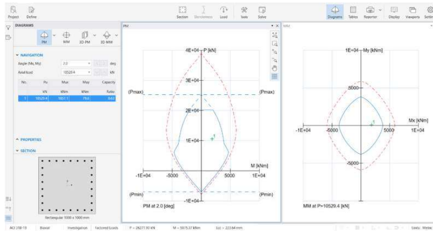
Gambar 4. 48 Diagram Interaksi Kolom K1 dengan aplikasi spColumn
