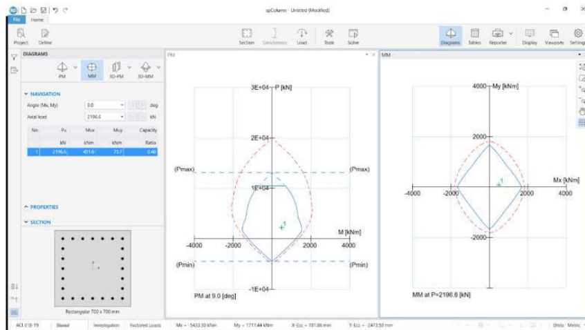
Gambar 4. 54 Diagram Interaksi Kolom K3 dengan aplikasi spColumn
