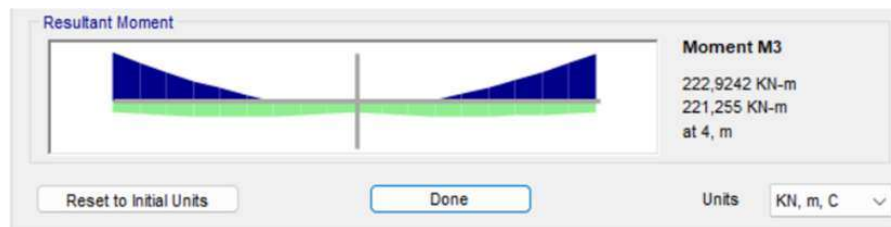
Gambar 4. 6 Output Momen Lapangan Arah Negatif Balok B1
