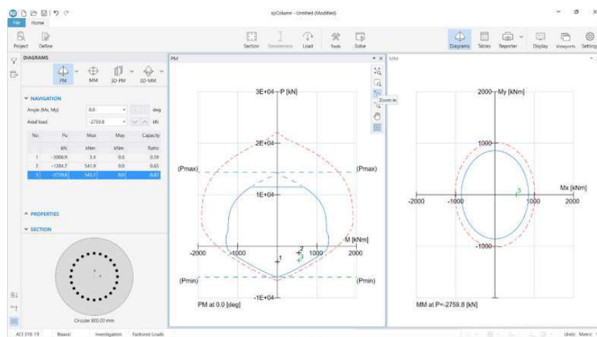
Gambar 4. 58 Gambar hasil menggunakan aplikasi SPColumn
