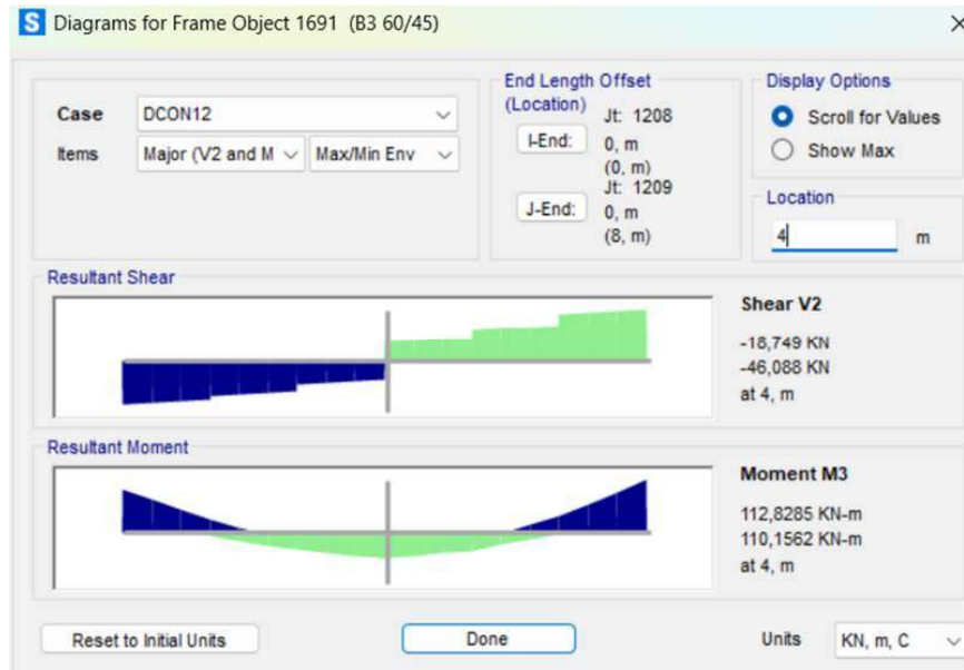
Gambar 4. 24 Output Momen Lapangan Arah Positif Balok B3
