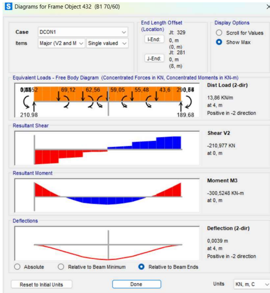
Gambar 4. 10 Output Gaya Geser Desain 1,2 D + 1,6 L Tumpuan Balok B1
