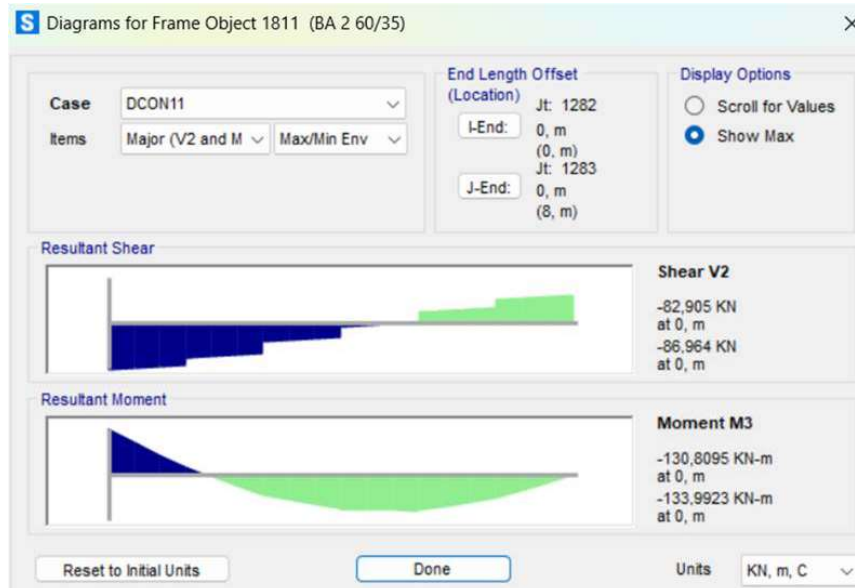
Gambar 4. 39 Output Momen Tumpuan Arah Negatif Balok BA1
