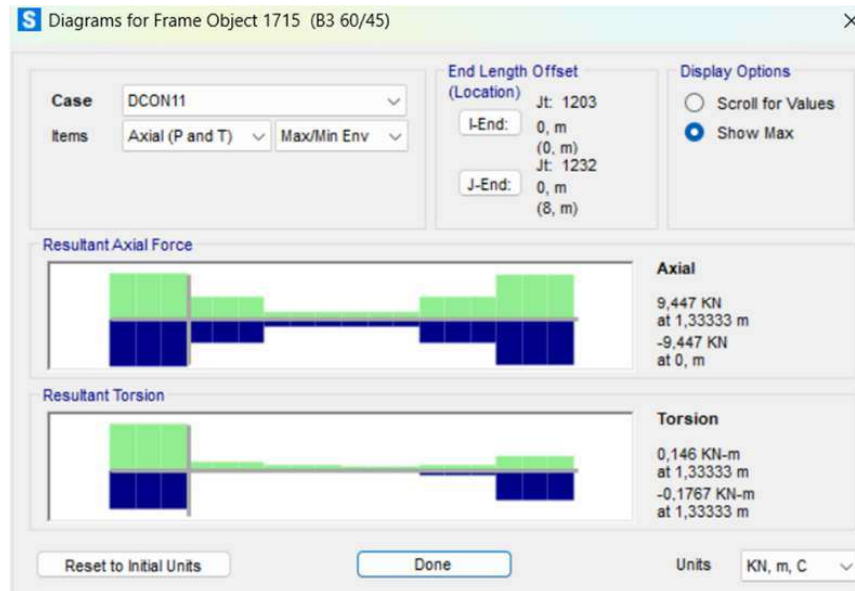
Gambar 4. 25 Output Gaya Aksial Balok B3
