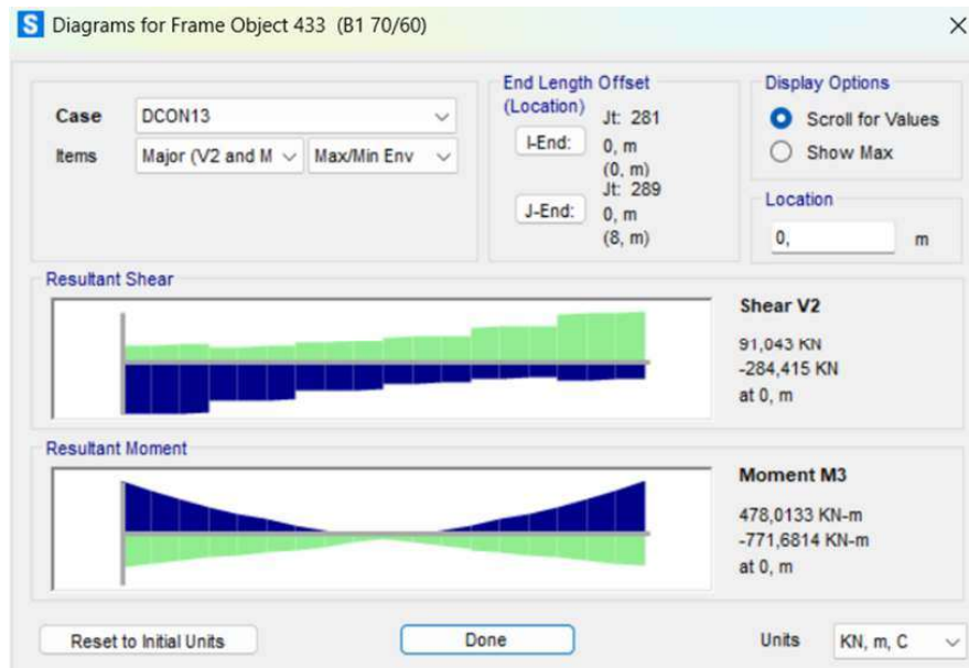
Gambar 4. 4 Output Momen Tumpuan Arah Positif Balok B1
