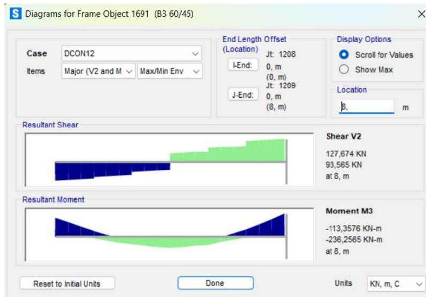
Gambar 4. 22 Output Momen Tumpuan Arah Positif Balok B3
