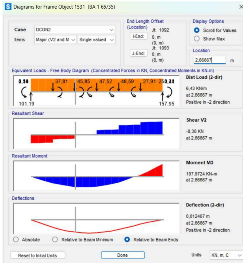
Gambar 4. 32 Output Momen Lapangan Arah Negatif Balok BA1
