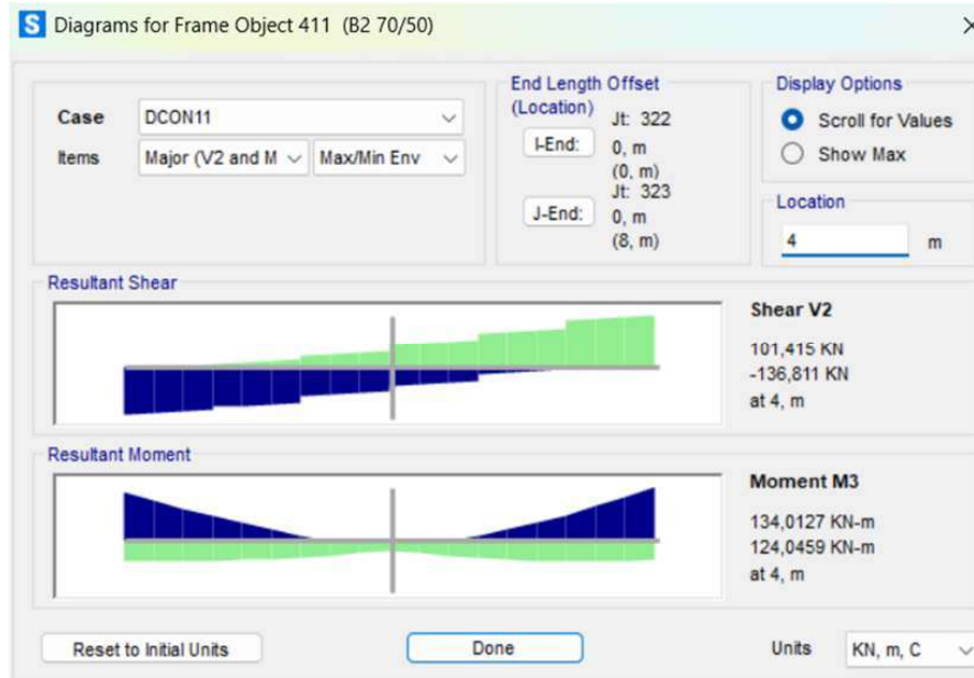
Gambar 4. 14 Output Momen Lapangan Arah Negatif Balok B2
