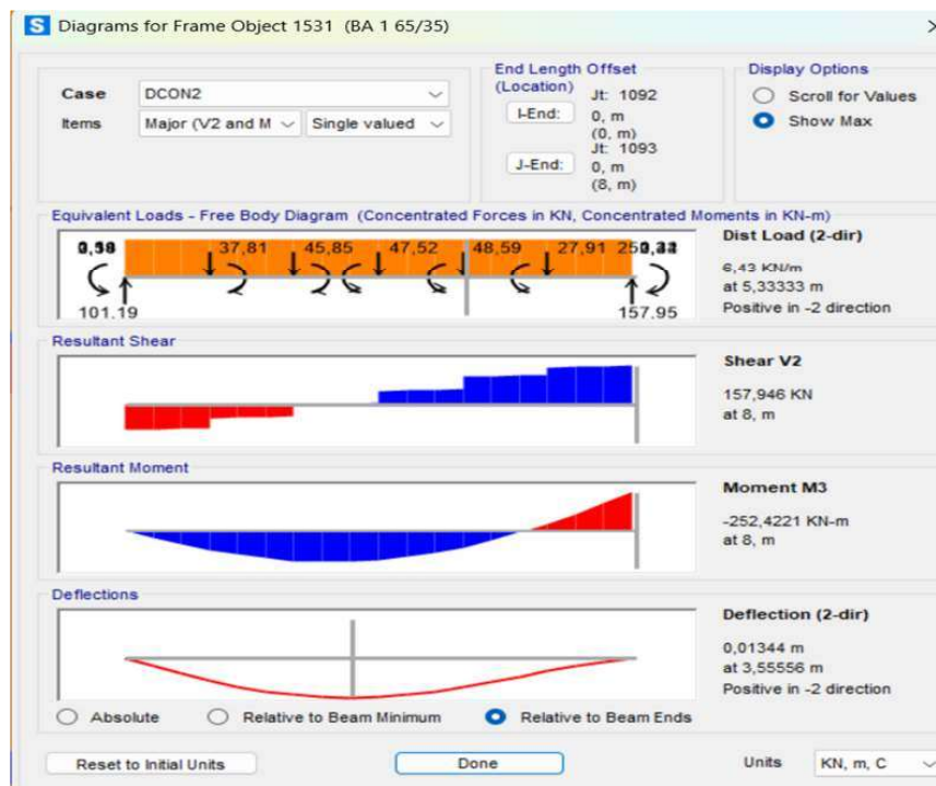
Gambar 4. 30 Output Momen Tumpuan Arah Negatif Balok BA1
