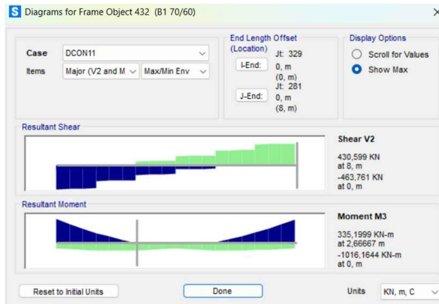
Gambar 4. 8 Output Gaya Geser Tumpuan Balok B1
