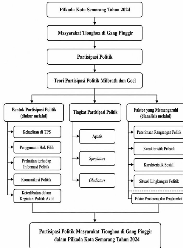
Gambar 1.1 Kerangka Berpikir
