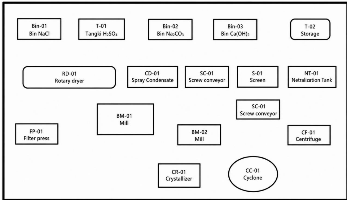
Gambar 2.6 Tata Letak Alat
