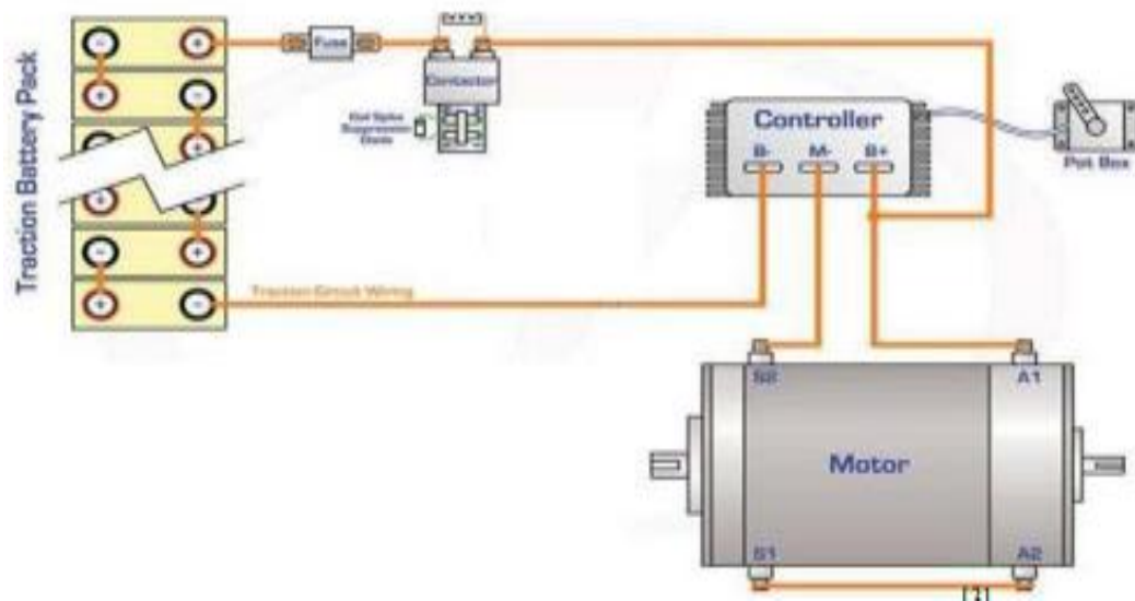
Gambar 2. 2 Sistem kelistrikan pada sepeda motor listrik
