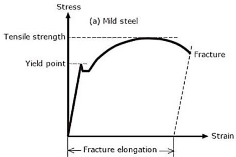
Gambar 2. 6 Grafik mild steel
