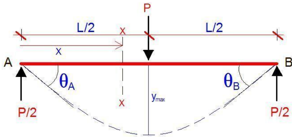
Gambar 2. 8 Defleksi balok sederhana
