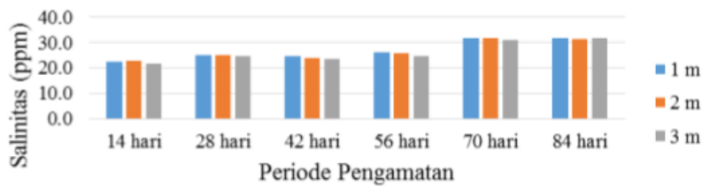
Gambar 2. Grafik perubahan salinitas air pada lebar saluran yang berbeda
