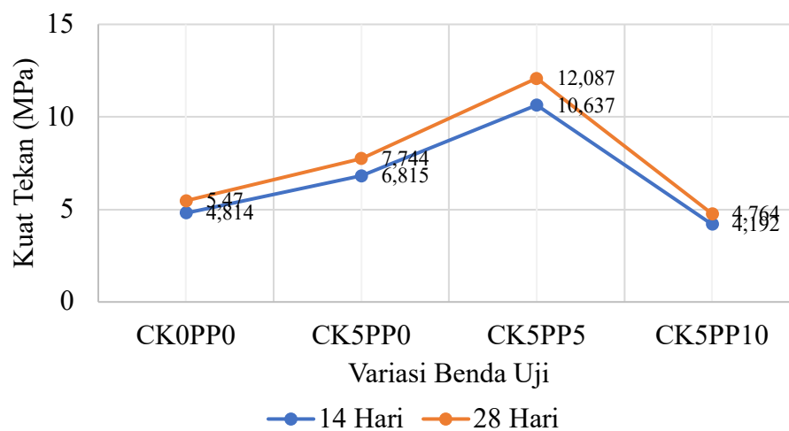
Gambar 4. 4 Grafik Hasil Kuat Tekan
