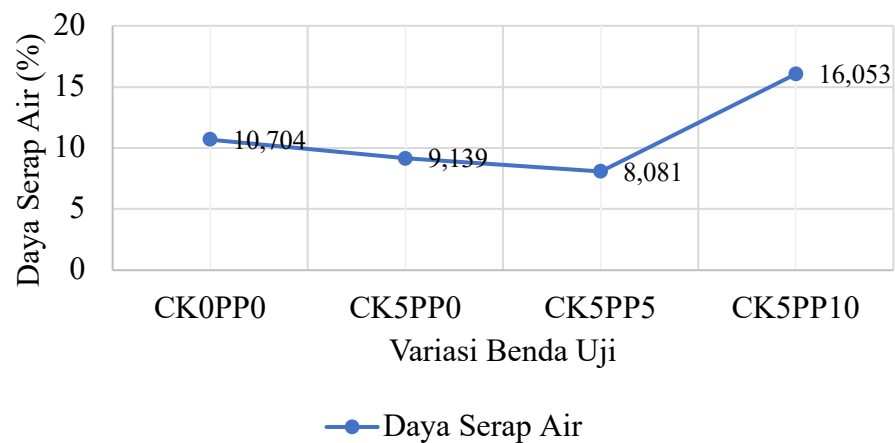
Gambar 4. 6 Grafik Hasil Daya Serap Air
