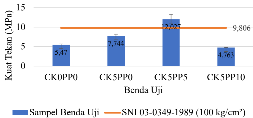
Gambar 4. 5 Grafik Hasil Kuat Tekan Pervariasi
