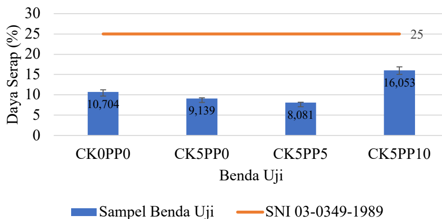
Gambar 4. 7 Grafik Hasil Daya Serap Air Pervariasi
