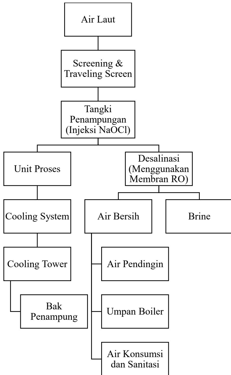
Gambar 4. 1. Diagram Alir Pengolahan Utilitas Air Pabrik Metil Metakrilat
