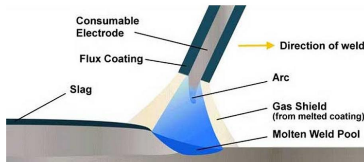
Gambar 2. 7 Proses pengelasan SMAW
