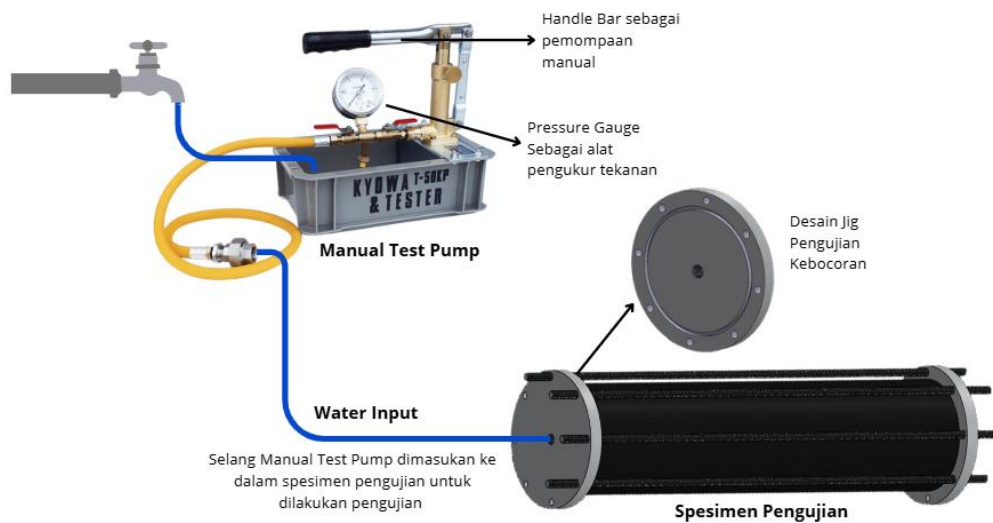
Gambar 2. 20 Pengujian hidrostatik
