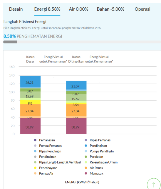
Gambar IV.16 Hasil Simulasi Energi Bangunan Eksisting pada EDGE APP
