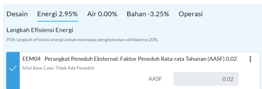
Gambar IV.76 Penerapan AASF Bangunan Redesain Perforated Panel pada EDGE APP
