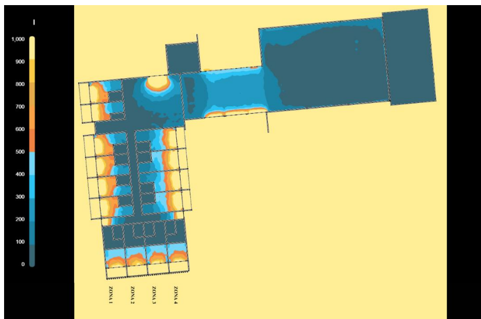
Gambar IV.58 Hasil Simulasi Fasad Fin Vertical Lantai 6 Pukul 12.00
