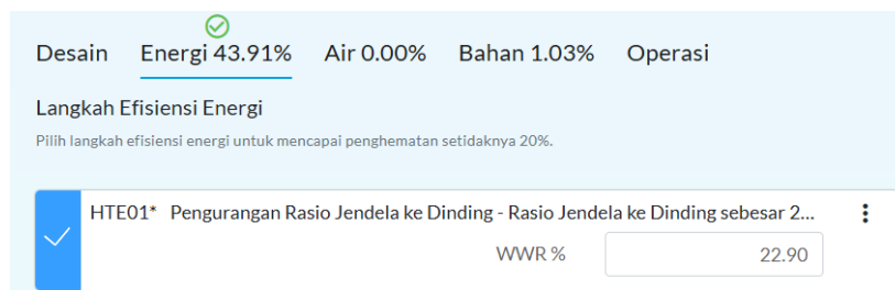
Gambar IV.113 Perhitungan WWR Bangunan Redesain Overhang Sunshading pada EDGE APP
