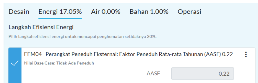
Gambar IV.41 Penerapan AASF Bangunan Redesain Fin Vertical pada EDGE APP
