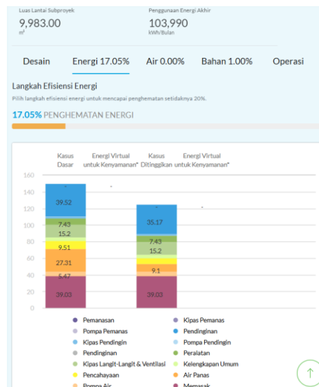
Gambar IV.39 Hasil Simulasi Energi Bangunan Redesain Fin Vertical pada EDGE APP
