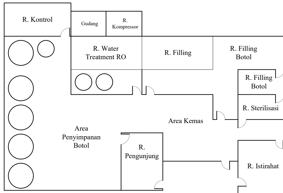
Gambar 2. 3 Layout Pabrik
