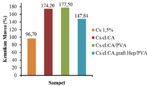
Gambar 3. Nilai serapan air membran
