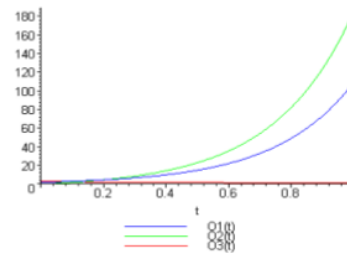
Gambar 3. Grafik O_1(t), O_2(t) dan O_3(t)
