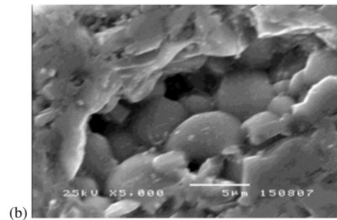
Gambar 4. Strukyut permukaan sampel Stoikiometri (a) dan Kelebihan 20% fraksi berat BaCO 3 (b) pada temperatur kalsinasi 1200°C selama 4 jam
