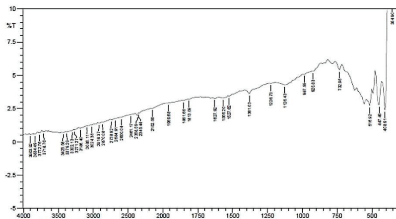
FIGURE 7. IR Spectra of CNT:MnO 2 75:25
