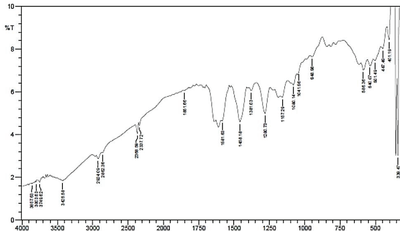
FIGURE 6. IR Spectra of CNT:MnO 2 50:50
