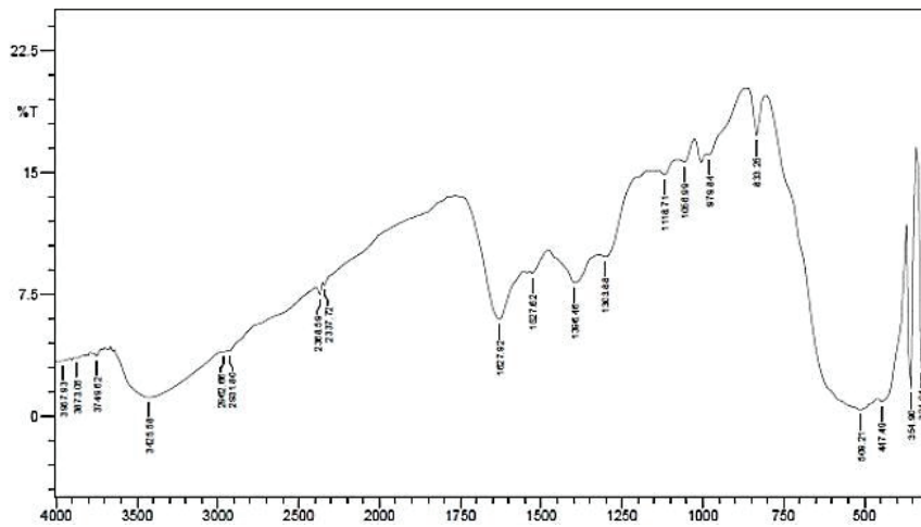
FIGURE 5. IR Spectra of CNT:MnO 2 25:75
