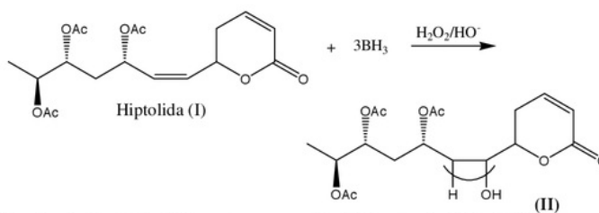
Gambar 3. Reaksi hidroborasi senyawa hiptolida menjadi alkohol turunannya
