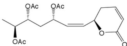
Gambar 2. Struktur senyawa hiptolida
