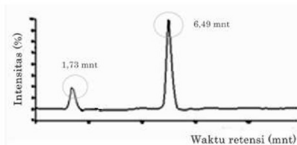
Gambar 5. Kromatogram produk hidroborasi
