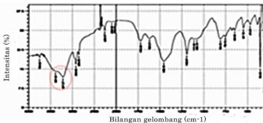
Gambar 4. Spektra infra merah produk hidroborasi
