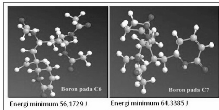
Gambar 7. Gambaran keadaan molekul untuk menerangkan regioselektivitas
