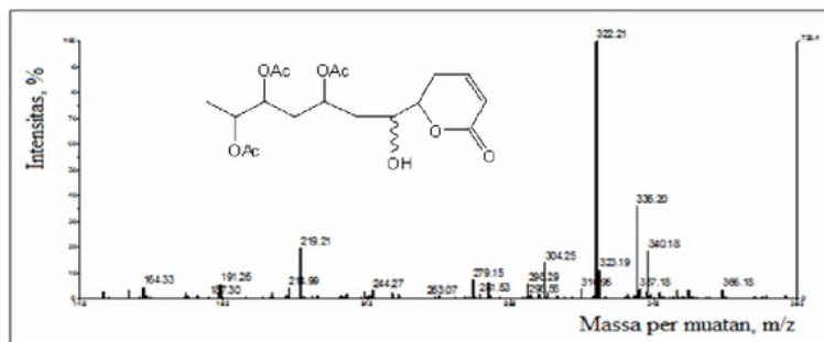
Gambar 6. Spectrogram massa produk hidroborasi dengan tr 1,73 menit
