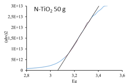
Gambar 4. Hasil Perhitungan Energi Celah Pita pada Pengukuran diffuse reflectance UV-Vis (DRS UV-Vis)
