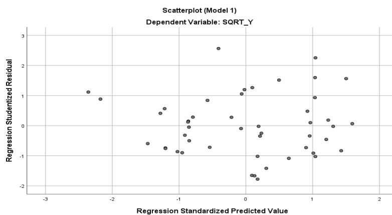
Gambar 5. Uji Heteroskedastisitas Model 1 (ROA)
