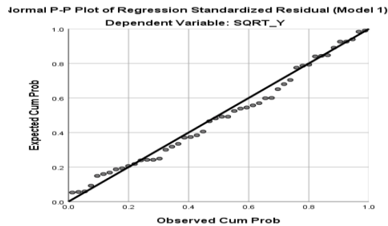
Gambar 2. Uji Normalitas Model 1 (ROA)
