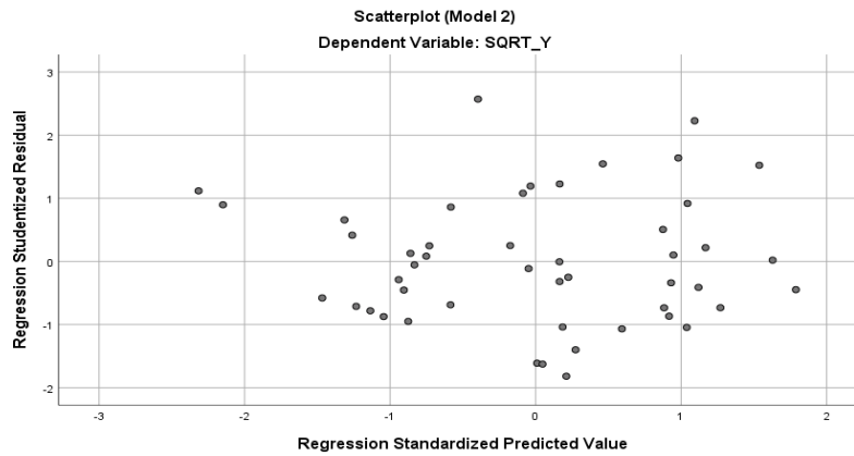
Gambar 6. Uji Heteroskedastisitas Model 2 (ROE)
