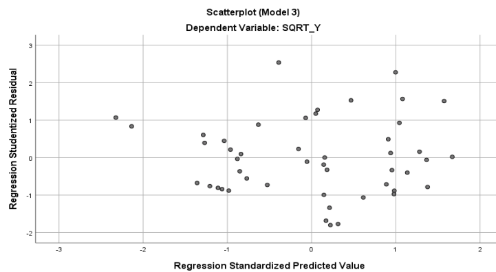
Gambar 7. Uji Heteroskedastisitas Model 3 (ROI)
