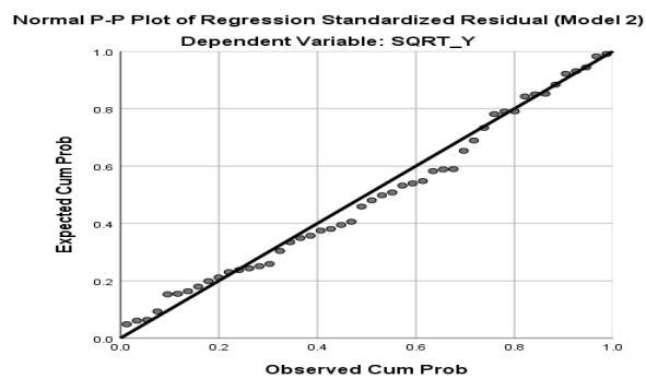
Gambar 3. Uji Normalitas Model 2 (ROE)
