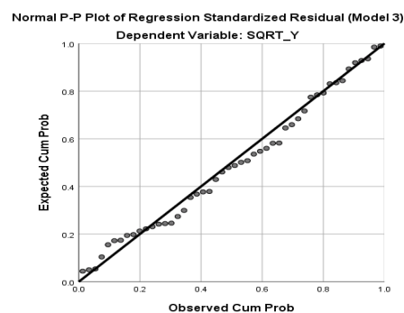
Gambar 4. Uji Normalitas Model 3 (ROI)
