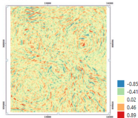
Gambar 5. Sebaran Korelasi Lokal Dengan Kelerengan
