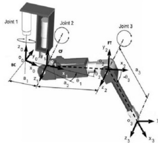
Gambar 4. Koordinat frames satu kaki hexapod robot [4].
