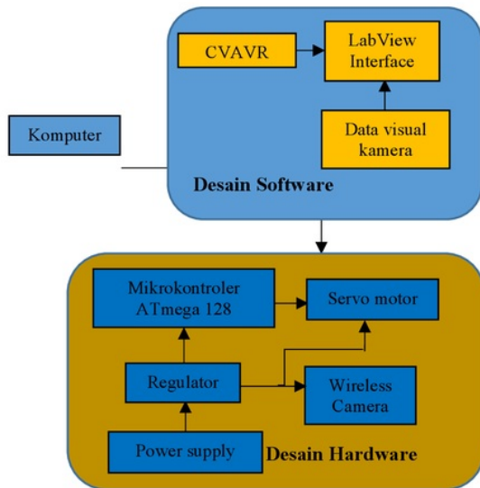
Gambar 2. Skema desain software dan hardware hexapod robot
