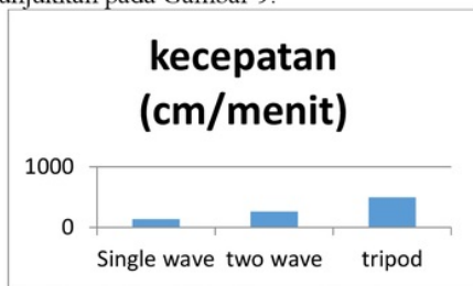
Gambar 9. Grafik hasil pengujian kecepatan
