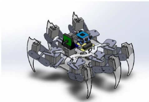
Gambar 1. Desain hexapod robot .
