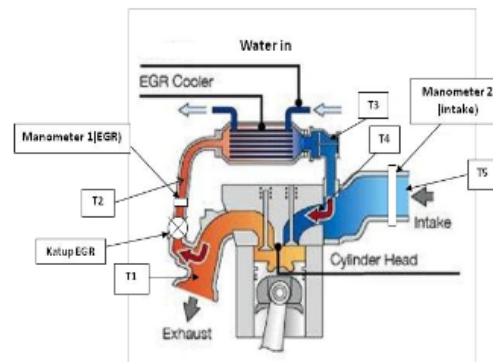
Gambar 1. Skema peralatan eksperimen
