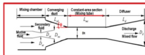
Gambar 4. Bentuk geometri steam ejector dalam penelitian
