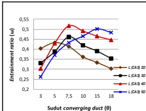
Gambar 5. Grafik hubungan antara sudut converging duct dan panjang constant-area section terhadap entrainment ratio steam ejector
