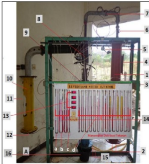
Gambar 2. Foto alat uji refrigerasi steam ejector
