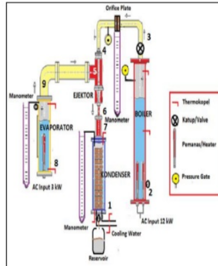
Gambar 3. Skema alat uji
