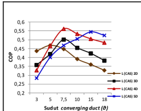
Gambar 6. Grafik hubungan antara sudut converging duct dan panjang constant-area section terhadap COP sistem refrigerasi steam ejector
