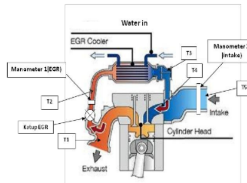
Gambar 1. Skema peralatan eksperimen
