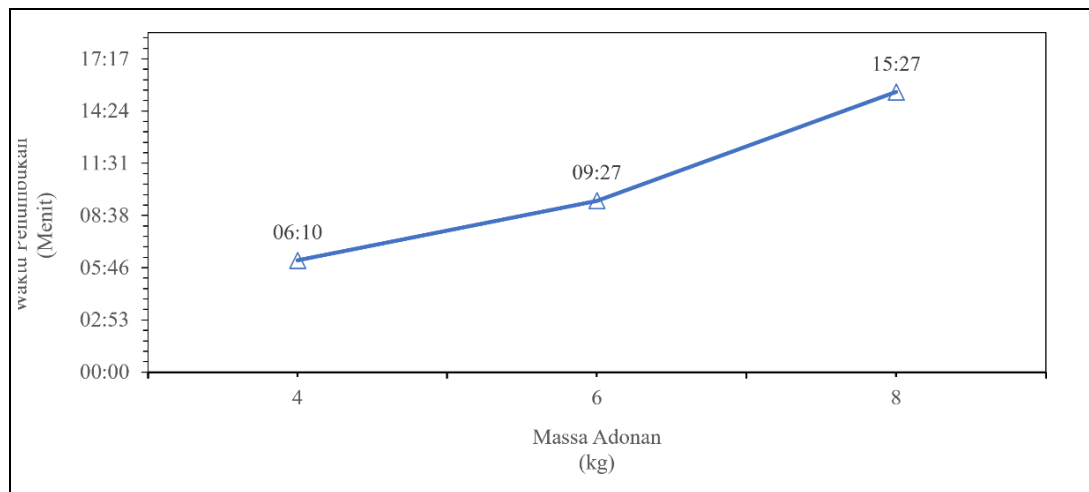
Gambar 4. 4 Grafik Pengujian Penumbukan dengan Putaran Motor 1000 RPM
