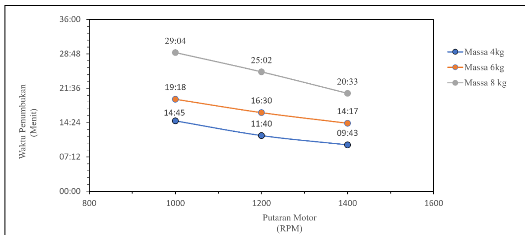
Gambar 4. 15 Grafik Hasil Perbandingan Waktu Produksi
