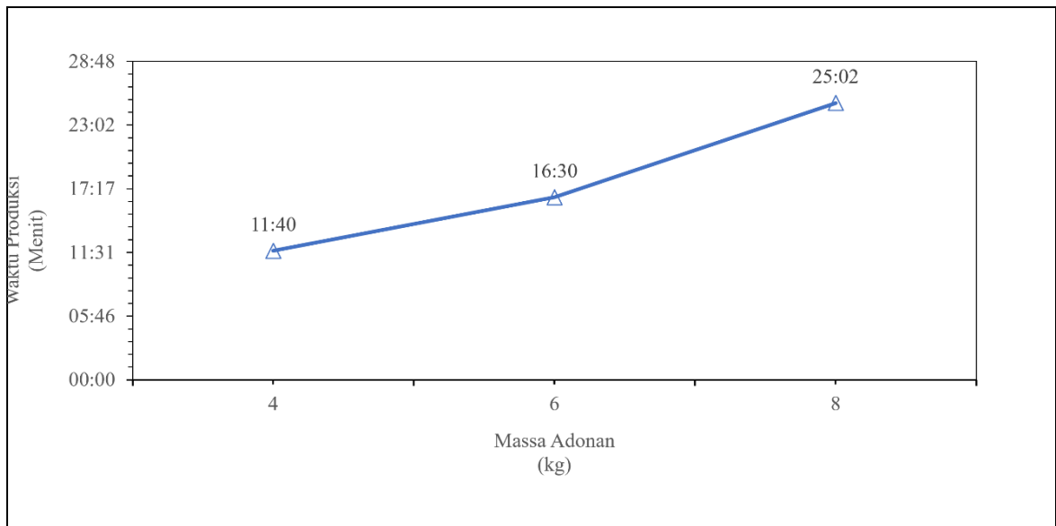
Gambar 4. 13 Grafik Pengujian Waktu Produksi dengan Putaran Motor Listrik 1200 RPM
