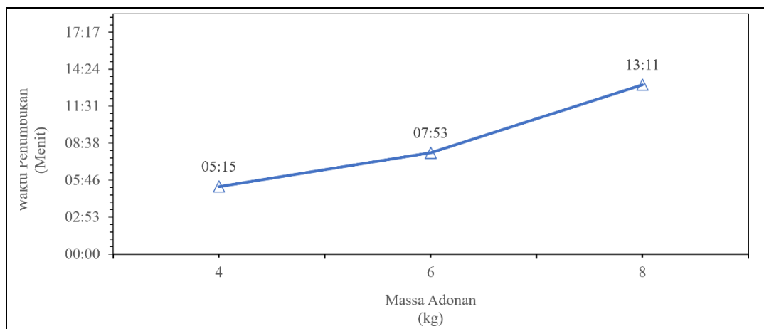
Gambar 4. 5 Grafik Pengujian Penumbukan dengan Putaran Motor Listrik 1200 RPM
