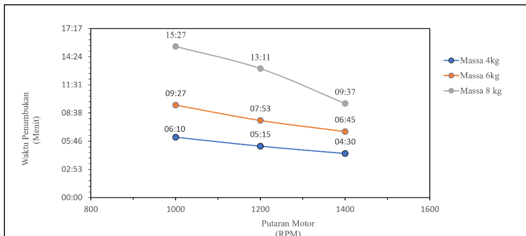
Gambar 4. 7 Grafik Hasil Perbandingan Waktu Penumbukan
