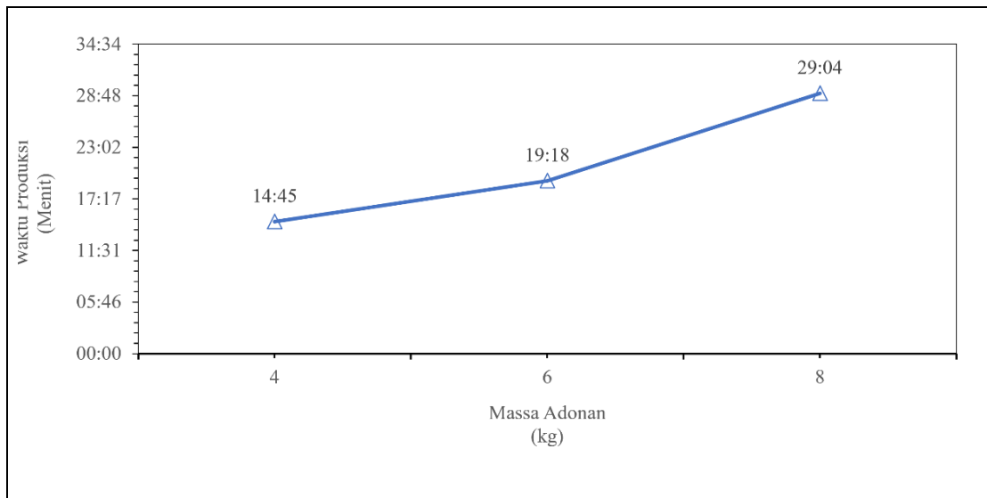
Gambar 4. 12 Grafik Pengujian Waktu Produksi dengan Putaran Motor Listrik 1000 RPM
