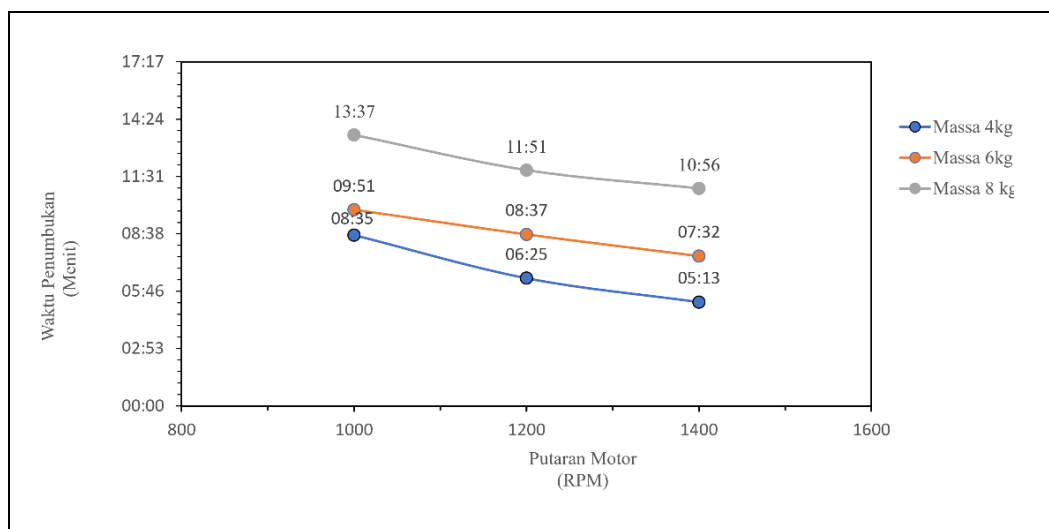
Gambar 4. 11 Grafik Hasil Perbandingan Waktu Pencetakan
