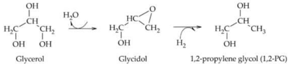
Gambar 1. 4 Mekanisme Esterifikasi-Hidrogenasi
