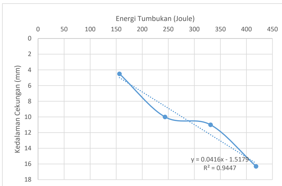
Gambar 4.10 Analisis penetrasi kedalaman residu terhadap energi tumbukan
