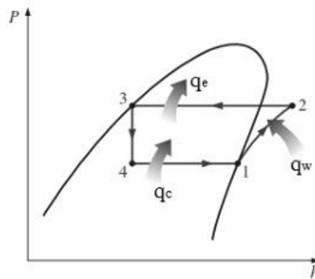
Gambar 2. 3 Siklus refrigrasi pada diagram P-h
