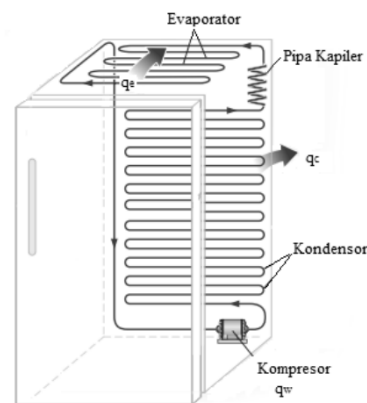
Gambar 2. 2 Siklus refrigasi pada mesin refrigasi
