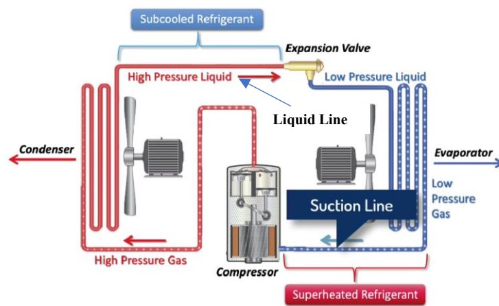
Gambar 2. 12 Skema sistem AC
