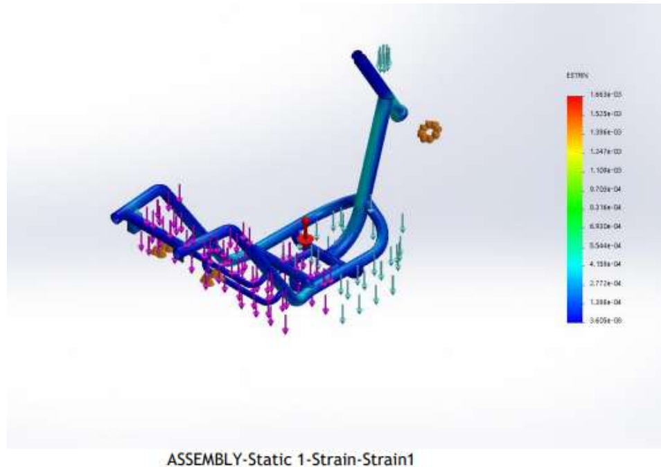
Gambar 2. 11 Contoh titik pembebanan pada rangka kendaraan roda tiga
