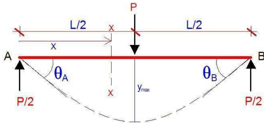
Gambar 2. 7 Defleksi balok sederhana
