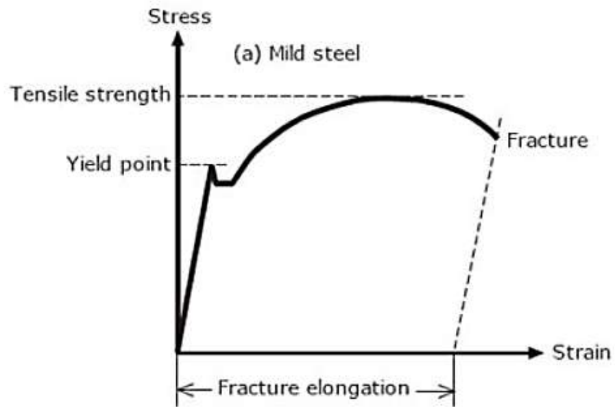
Gambar 2. 5 Grafik mild steel Sumber : Callister, W. D., & Rethwisch, D. G., 2020
