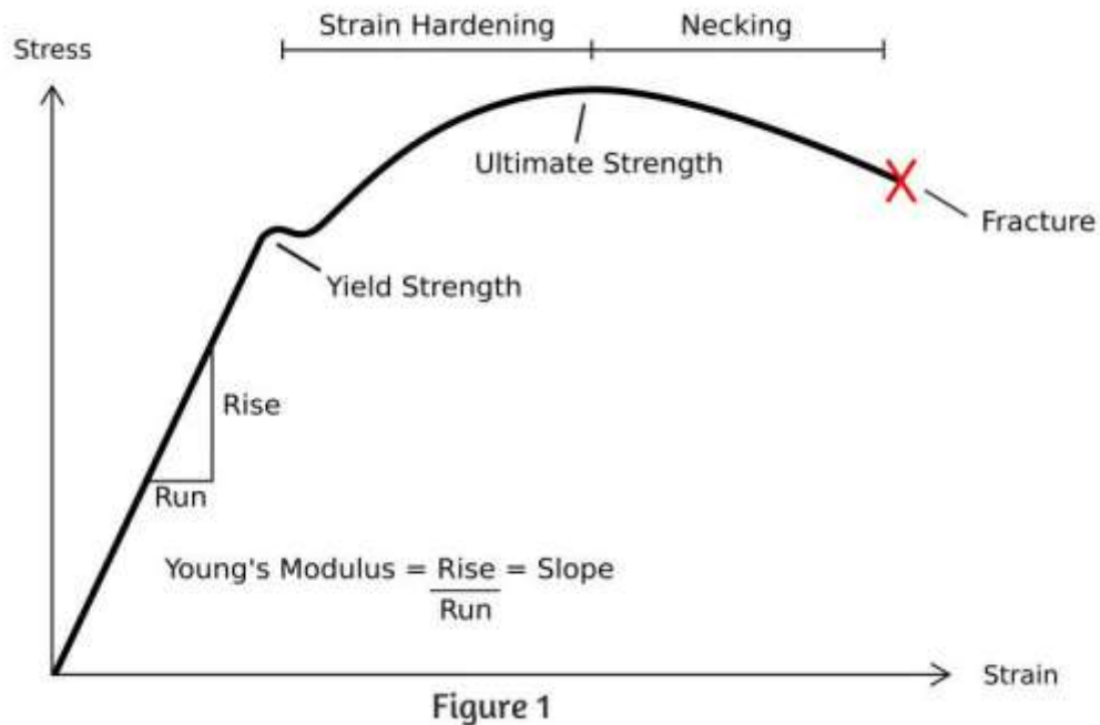
Gambar 2. 4 Grafik yield point atau batas luluh
