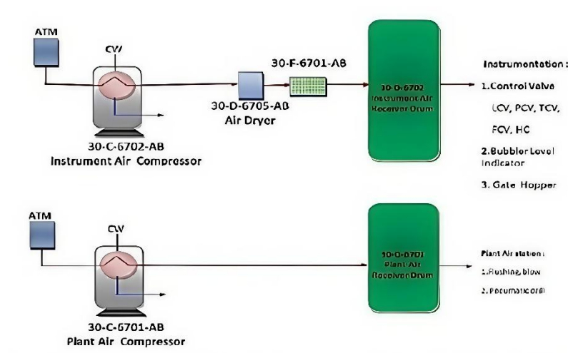
Gambar 4.3 Diagram Alir Pengadaan Udara Tekan
