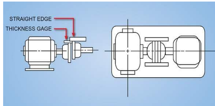
Gambar 2. 7 Metode straightedges
