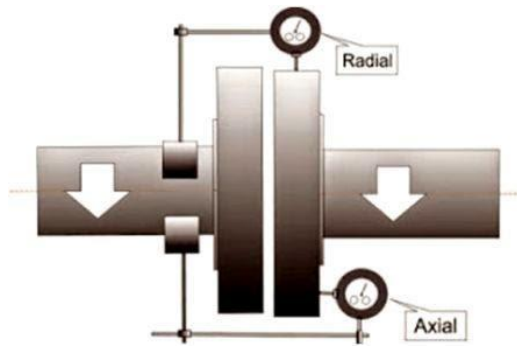
Gambar 2. 9 Memutar kedua poros
