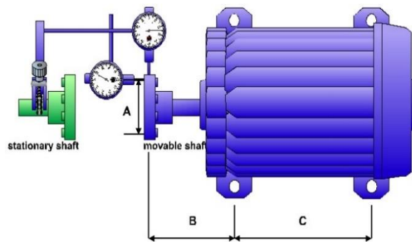
Gambar 2. 10 Sketsa pengaplikasian formula matematis
