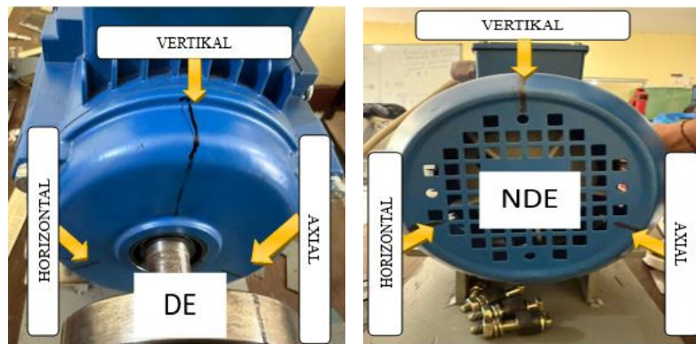
Gambar 2. 19 Bagian- bagian NDE dan DE yang diukur
