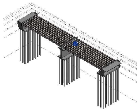
Gambar 4. 49 Pekerjaan Diafragma
