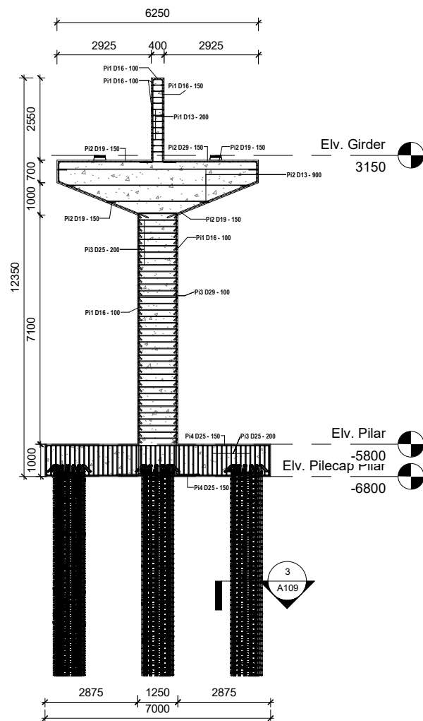
1 Detail Pilar 1 : 100
