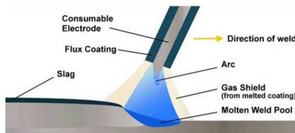
Gambar 2. 7 Proses pengelasan SMAW
