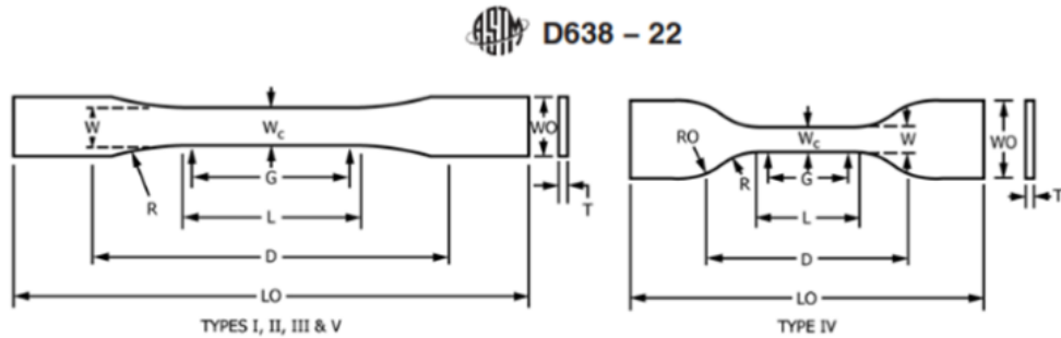
Gambar 2. 18 Spesimen uji tarik
