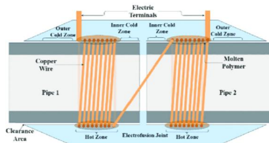
Gambar 2. 11 Proses pengelasan electrofusion
