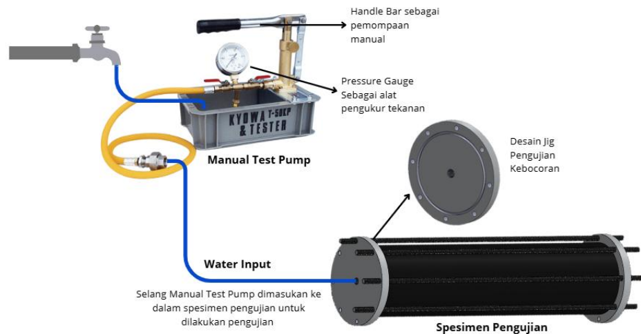
Gambar 2. 20 Pengujian hidrostatik
