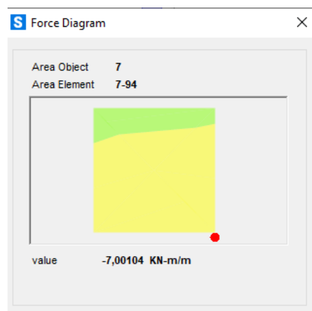
Gambar 4. 25 Momen Tumpuan Arah Y
