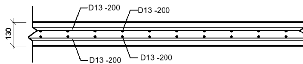
3 DETAIL P13 1 : 20
