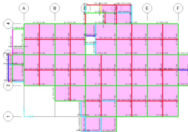
Gambar 4. 7 Permodelan Balok dan Pelat Lantai 2
