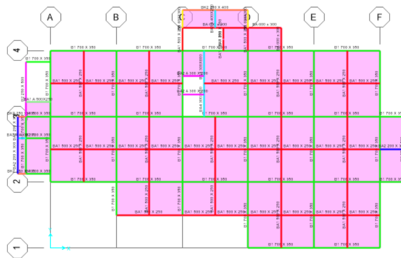
Gambar 4. 8 Permodelan Balok dan Pelat Lantai 3
