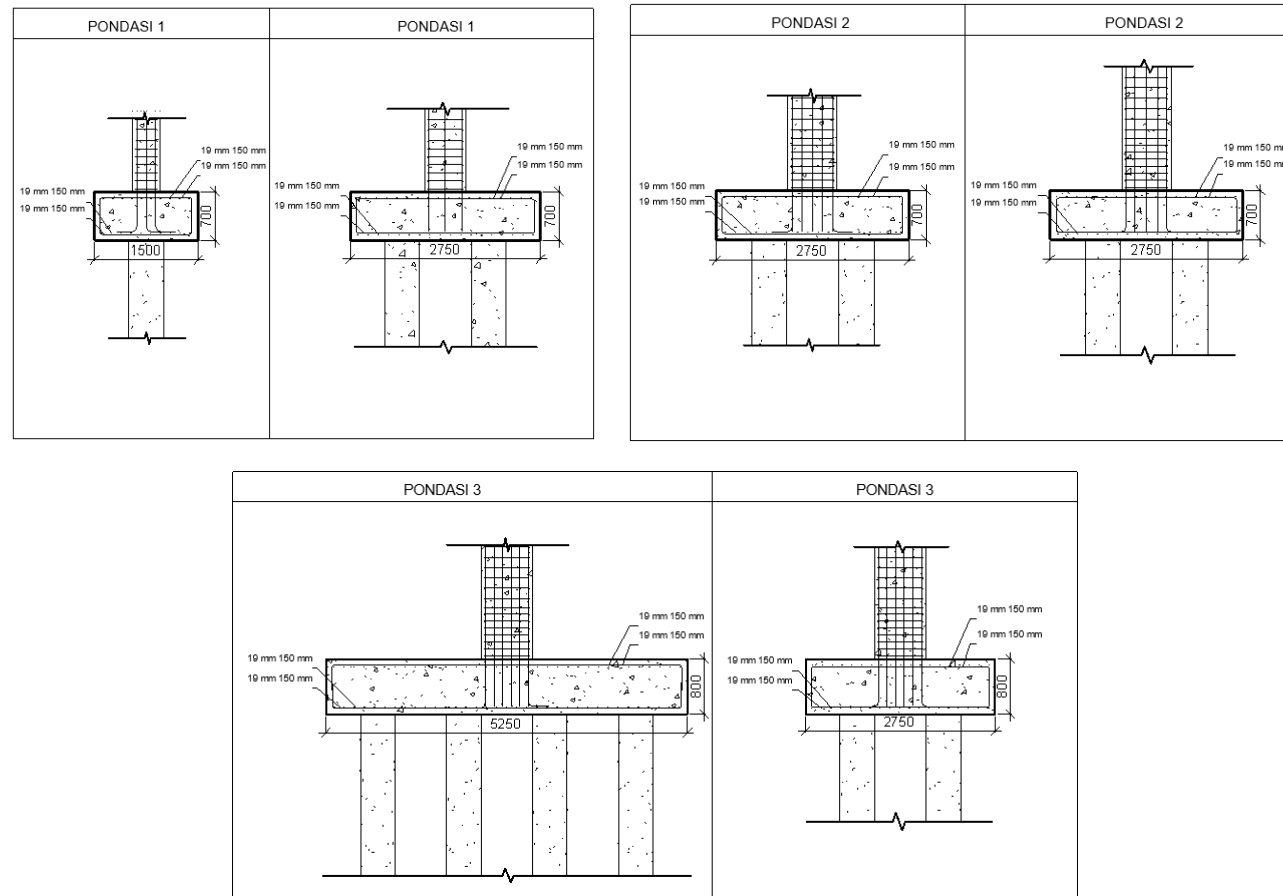
Gambar 4. 27 Penulangan Pile Cap
