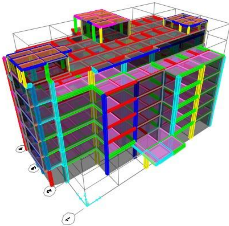
Gambar 4. 14 Permodelan Struktur pada SAP 2000 Sumber: Analisa Penulis, 2025
