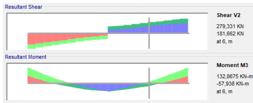
Gambar 4. 18 Output Gaya Dalam Area Lapangan
