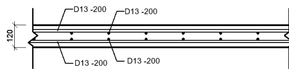
1 DETAIL P10 1 : 20
