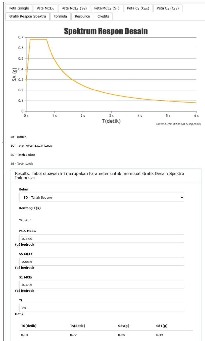
Gambar 4.5 Spektrum Respon Desain (Sumber: rsa.ciptakarya.pu.go.id/2021, 2025)
