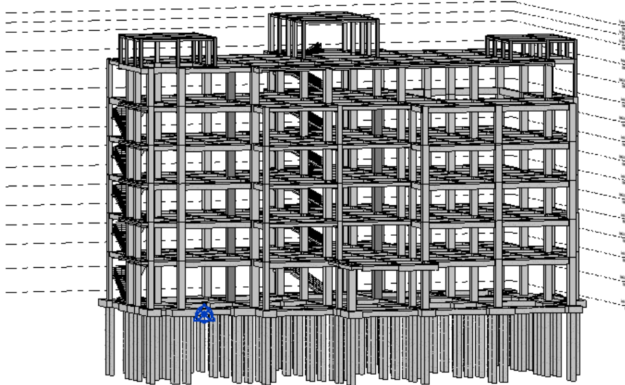
Gambar 4. 28 Permodelan 3D Elemen Struktur dengan Revit
