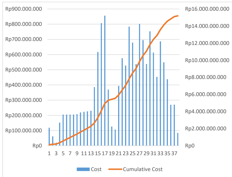
Grafik 4. 1 Kurva S Pembangunan Gedung ICT UNDIP
