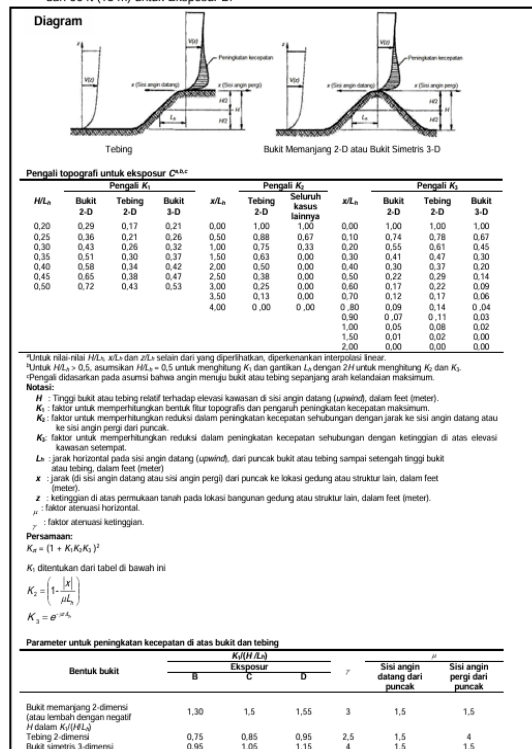
Gambar 26.8-1 - Faktor topografi, K_a
