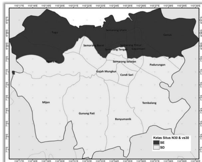
Gambar 4. 4 Peta Klasifikasi Situs Kota Semarang
