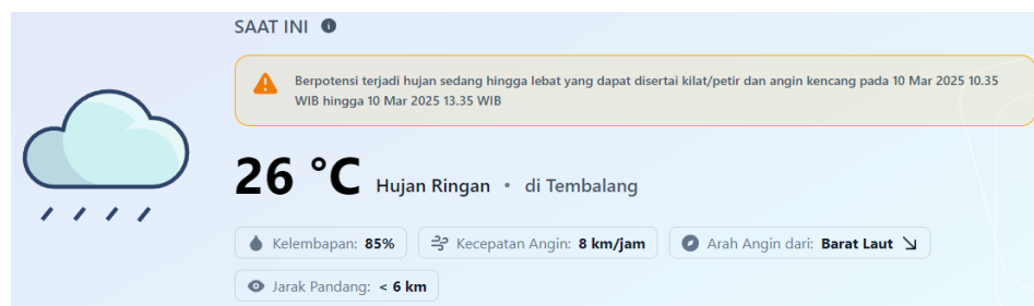
Gambar 4. 1 Kecepatan Angin Daerah Tembalang, Kabupaten Semarang Tahun 2025
