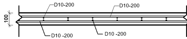
1 DETAIL P10 1 : 20
