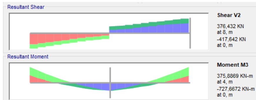
Gambar 4. 17 Output Gaya Dalam Area Tumpuan
