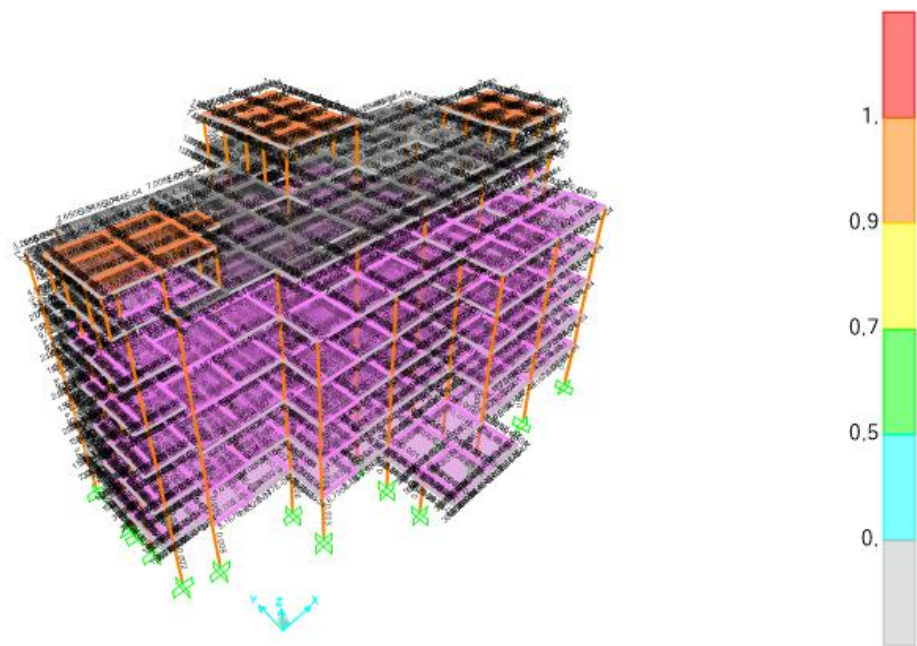
Gambar 4. 15 Hasil Analisa Rasio Batang
