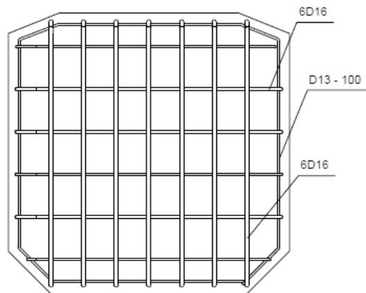
Gambar 4. 49 Detail Penulangan Diafragma
