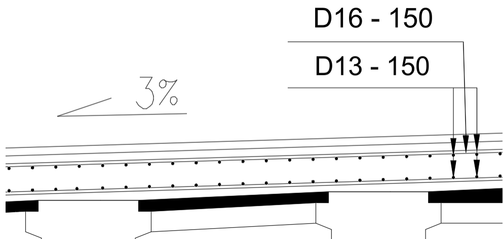
Gambar 4. 31 Detail Penulangan Pelat Lantai
