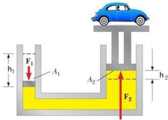
Gambar 2. 5 Ilustrasi Prinsip Hukum Pascal
