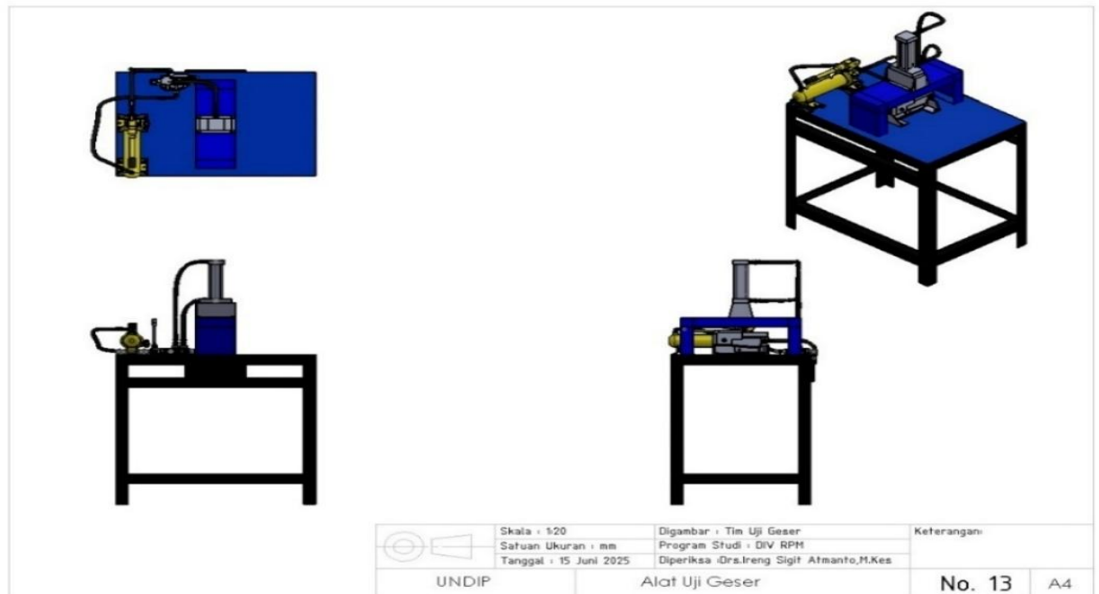
Gambar 3. 23 Desain alat uji geser
