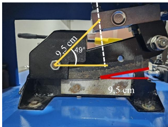
Gambar 3. 2 Pisau pemotong
