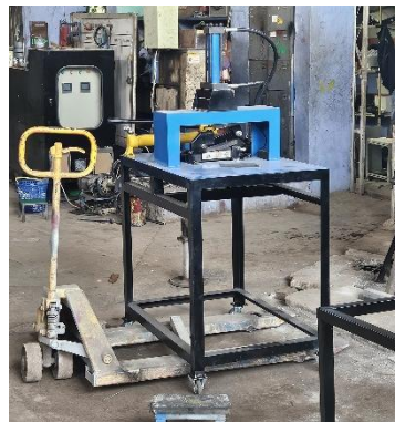
Gambar 3. 29 Hasil fabrikasi
