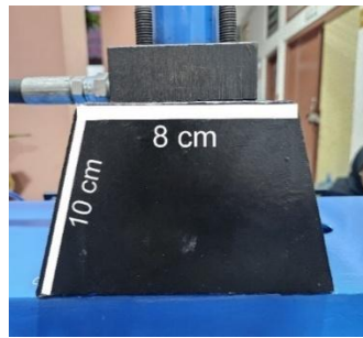
Gambar 3. 4 Dudukan silinder
