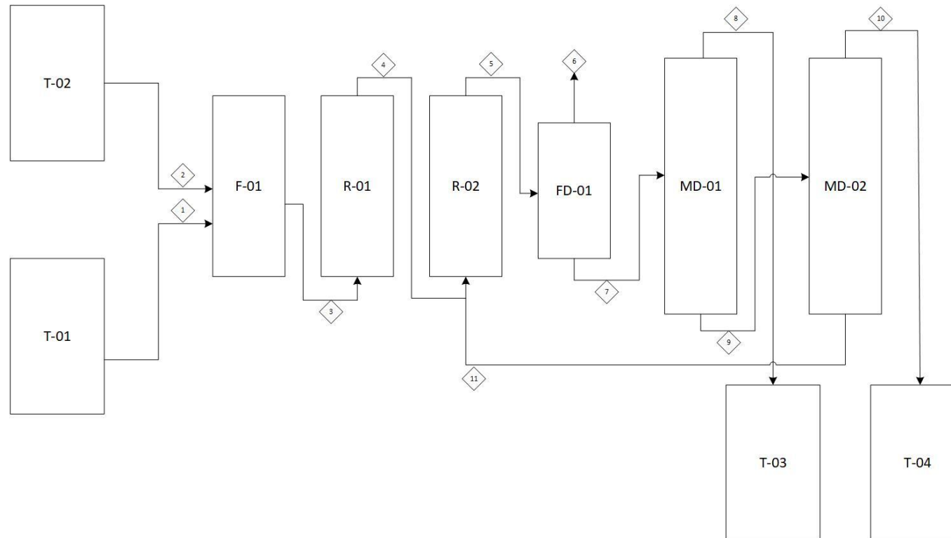
Gambar 2.20. Diagram alir neraca massa Pabrik Isopropil Benzena (Cumene) dengan kapasitas 50.000 ton/tahun
