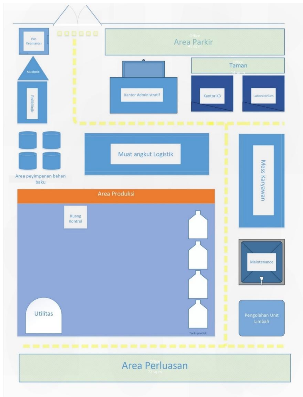
Gambar 2. 22. Layout Pabrik Isopropil Benzene (Cumene) dengan kapasitas 50.000 ton/tahu
