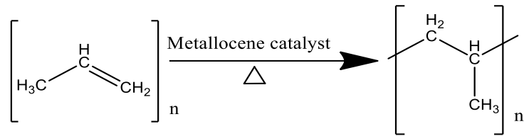
Gambar 2. 5. Reaksi polimerisasi propilena menjadi polipropilena
