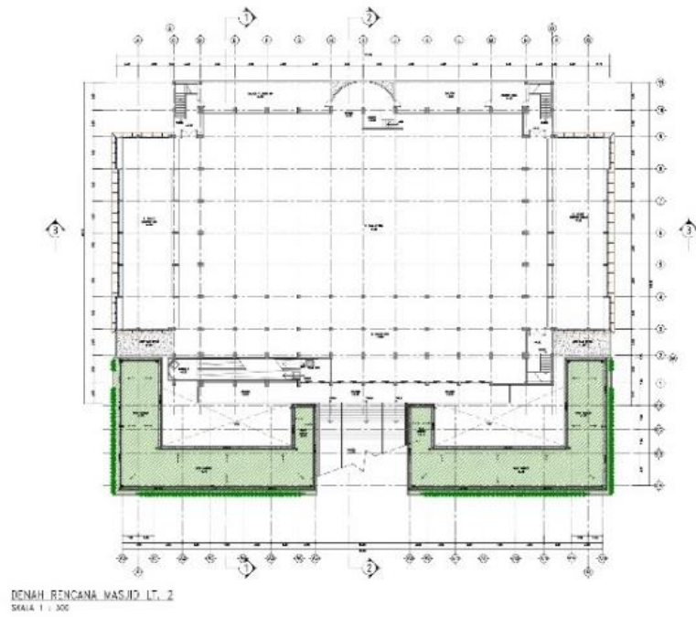
Gambar 3.6 : Denah Eksisting Masjid Raya Baiturrahman Semarang Jawa Tengah Lantai 2
