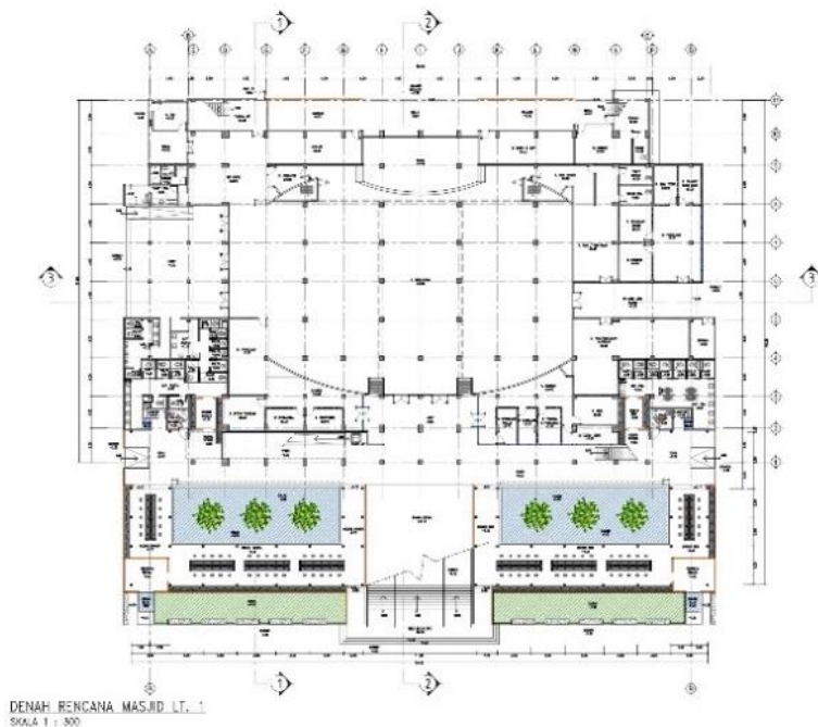
Gambar 3.5 : Denah Eksisting Masjid Raya Baiturrahman Semarang Jawa Tengah Lantai 1
