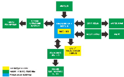
Gambar 3. Blok Diagram Keseluruhan
