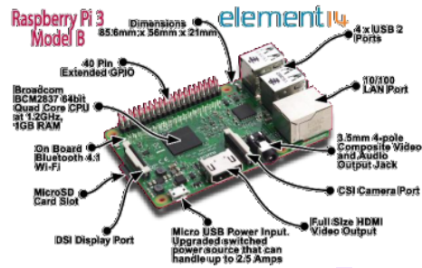
Gambar 1 Bentuk fisik Raspberry Pi 3 B Python
