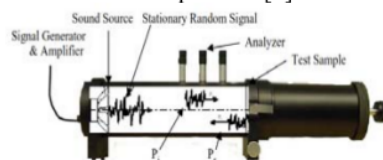
Gambar 2.1 Tabung impedansi dua mikrofon.
