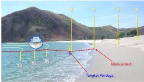
Gambar 1 Metode Pengukuran Garis Pantai Terestris (BIG, 2017)
