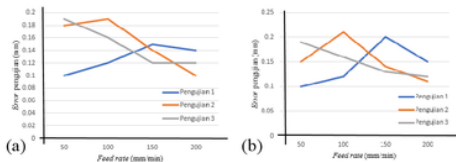
Gambar 8. Optimasi gerakan full-step untuk (a) sumbu X; (b) sumbu Y.
