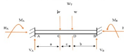
Gambar 2. Diagram benda bebas satu poros terpusat.
