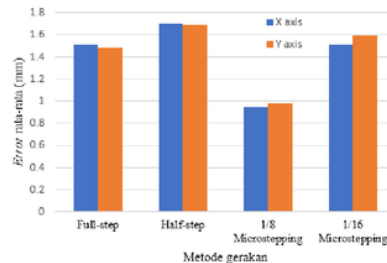
Gambar 12. Grafik perbandingan metode gerakan.
