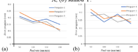
Gambar 9. Optimasi gerakan half step untuk (a) sumbu X; (b) sumbu Y.
