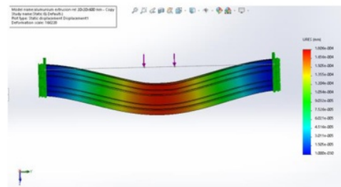
Gambar 3. Nilai defleksi pada poros sumbu X.
