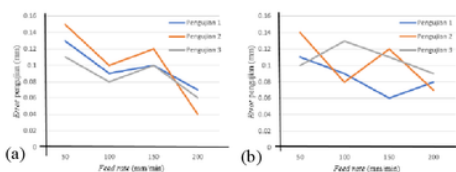
Gambar 10. Optimasi gerakan 1/8 micro stepping untuk (a) sumbu X; (b) sumbu Y.
